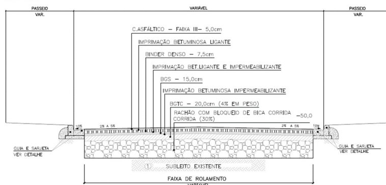
DETALHE 1: SEÇÃO-TIPO DO PAVIMENTO – "A-A" TRÁFEGO PESADO ESC. 1:50
