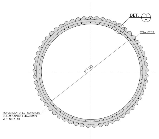
"TUNNEL LINER" Ø3,00m (ACABADO) PROJETADO ESCALA 1:25
