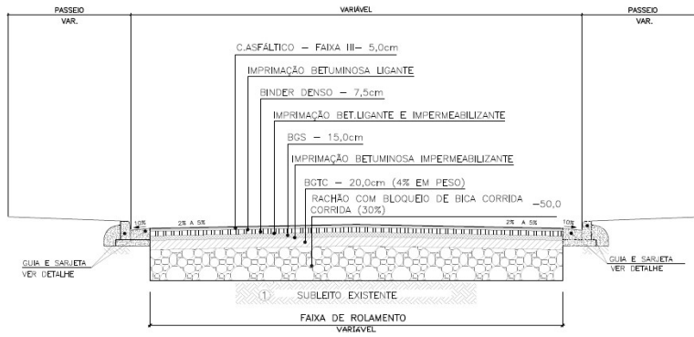
DETALHE 1: SEÇÃO-TIPO DO PAVIMENTO – "A-A" TRÁFEGO PESADO ESC. 1:50
