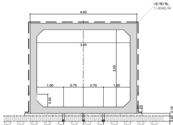
SEÇÃO TIPO GALERIA RETANGULAR FECHADA EM CONCRETO SEÇÃO 3,50mx3,00m ESCALA 1:50
