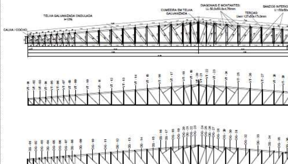
DETALHAMENTO DO PÓRTICO Escala: 1:100
