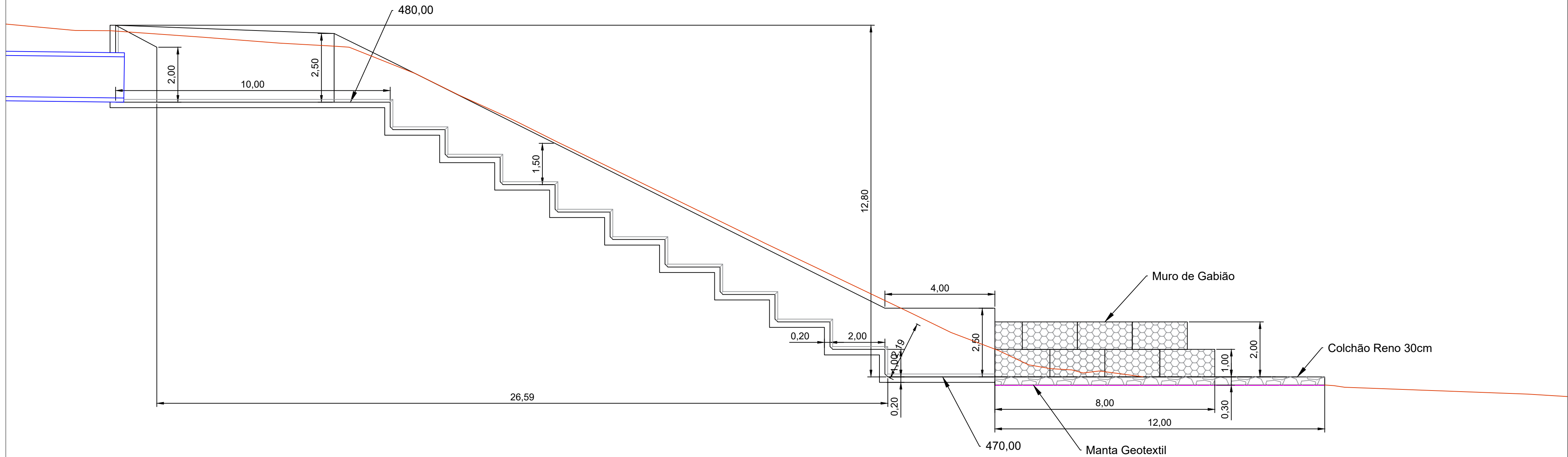
Escada dissipadora
