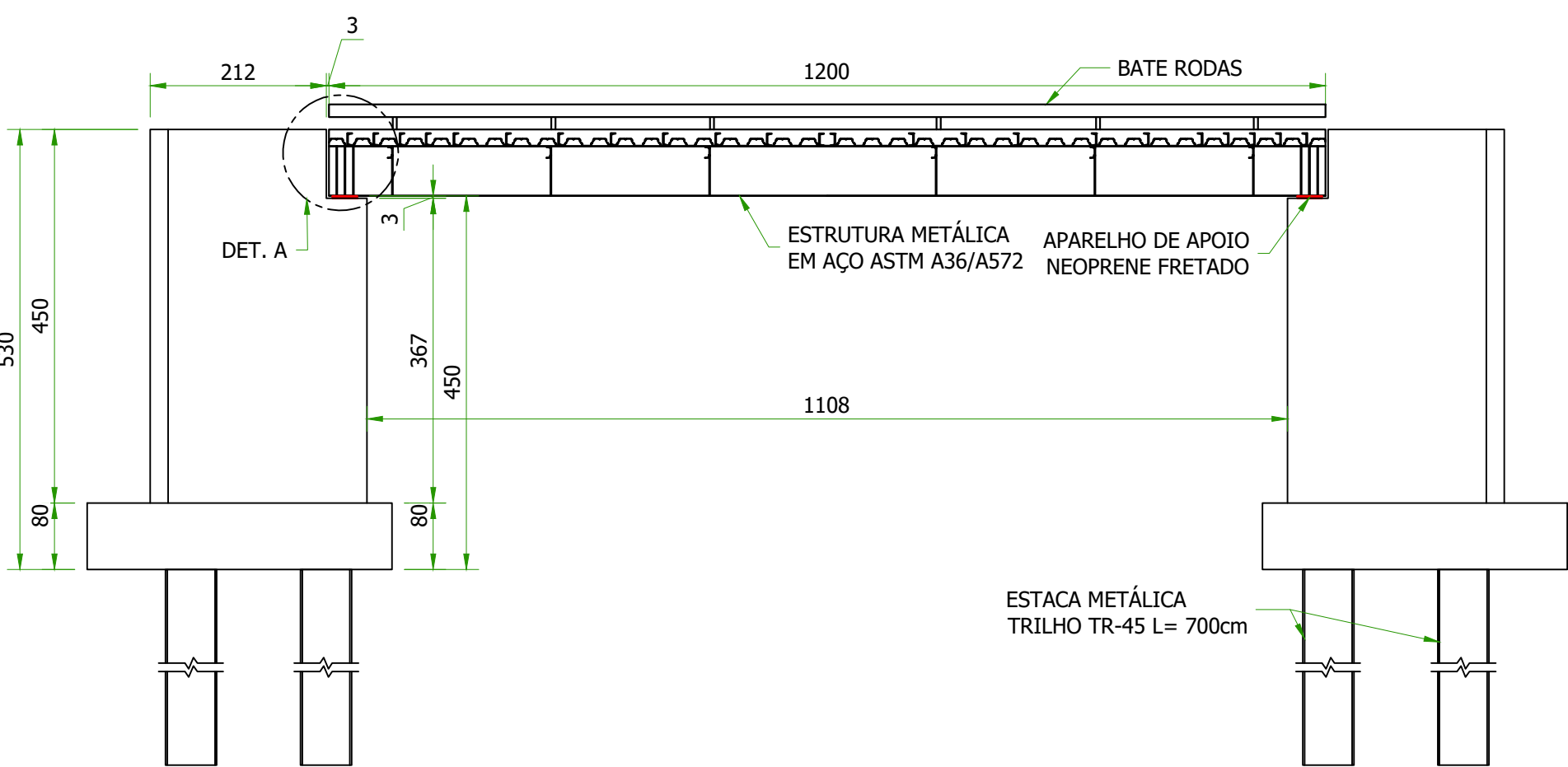
SEÇÃO LONGITUDINAL ESCALA 1:75
