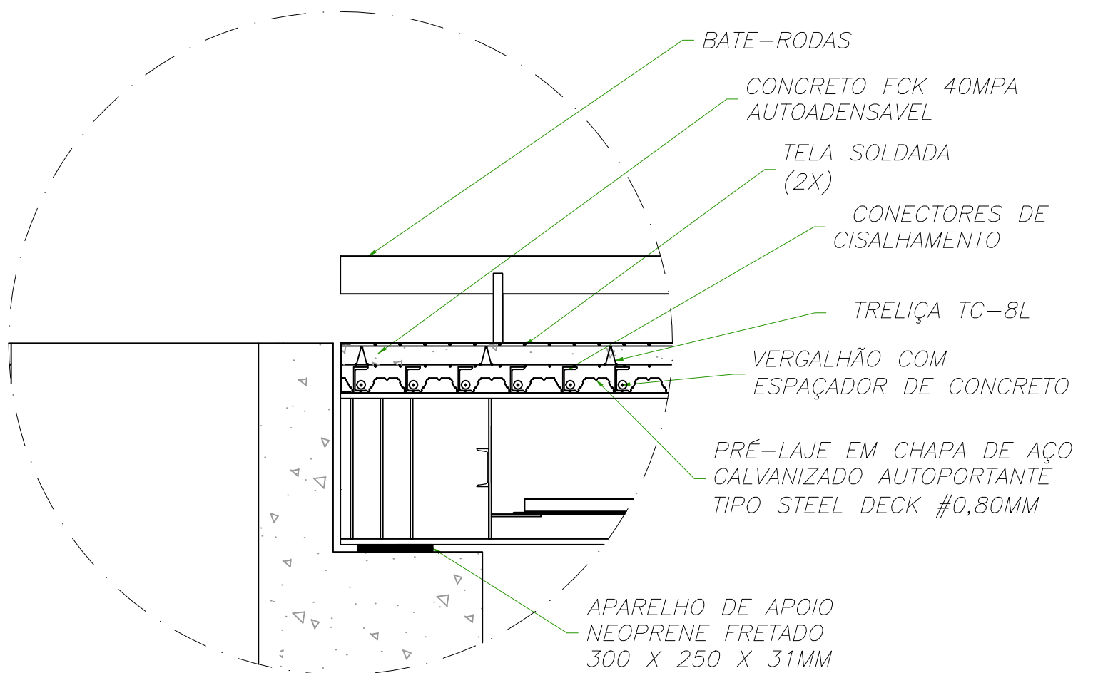
DETALHE A SEM ESCALA
