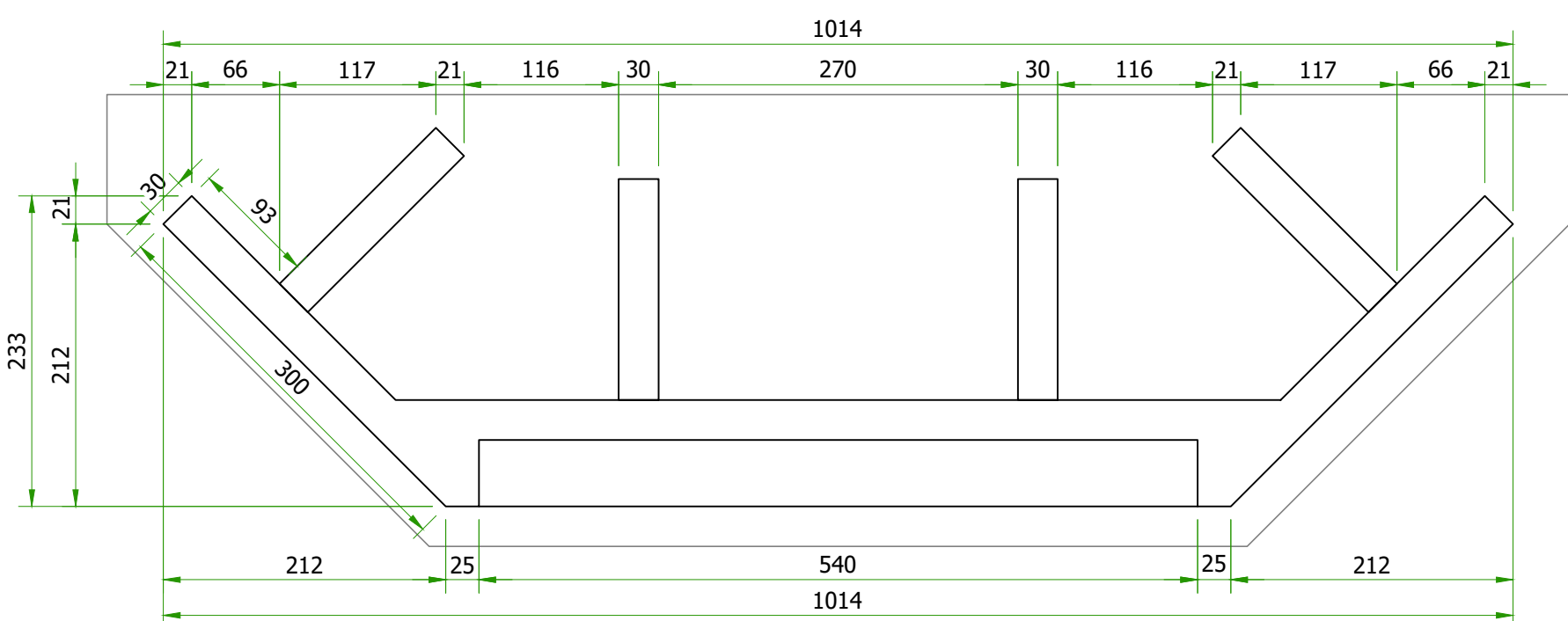
PLANTA BAIXA DA CABECEIRA ESCALA 1:50
