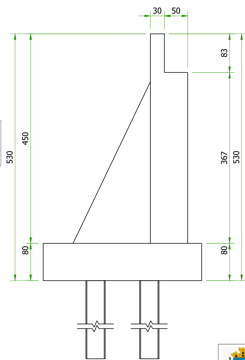
CORTE A-A
