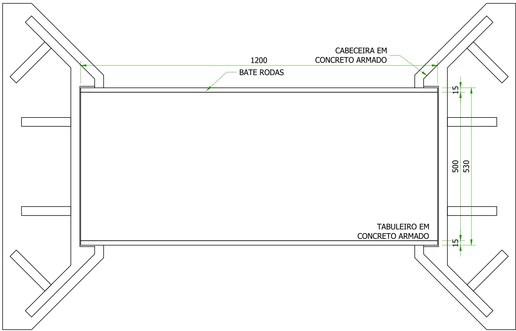
PLANTA DO TABULEIRO ESCALA 1:75
