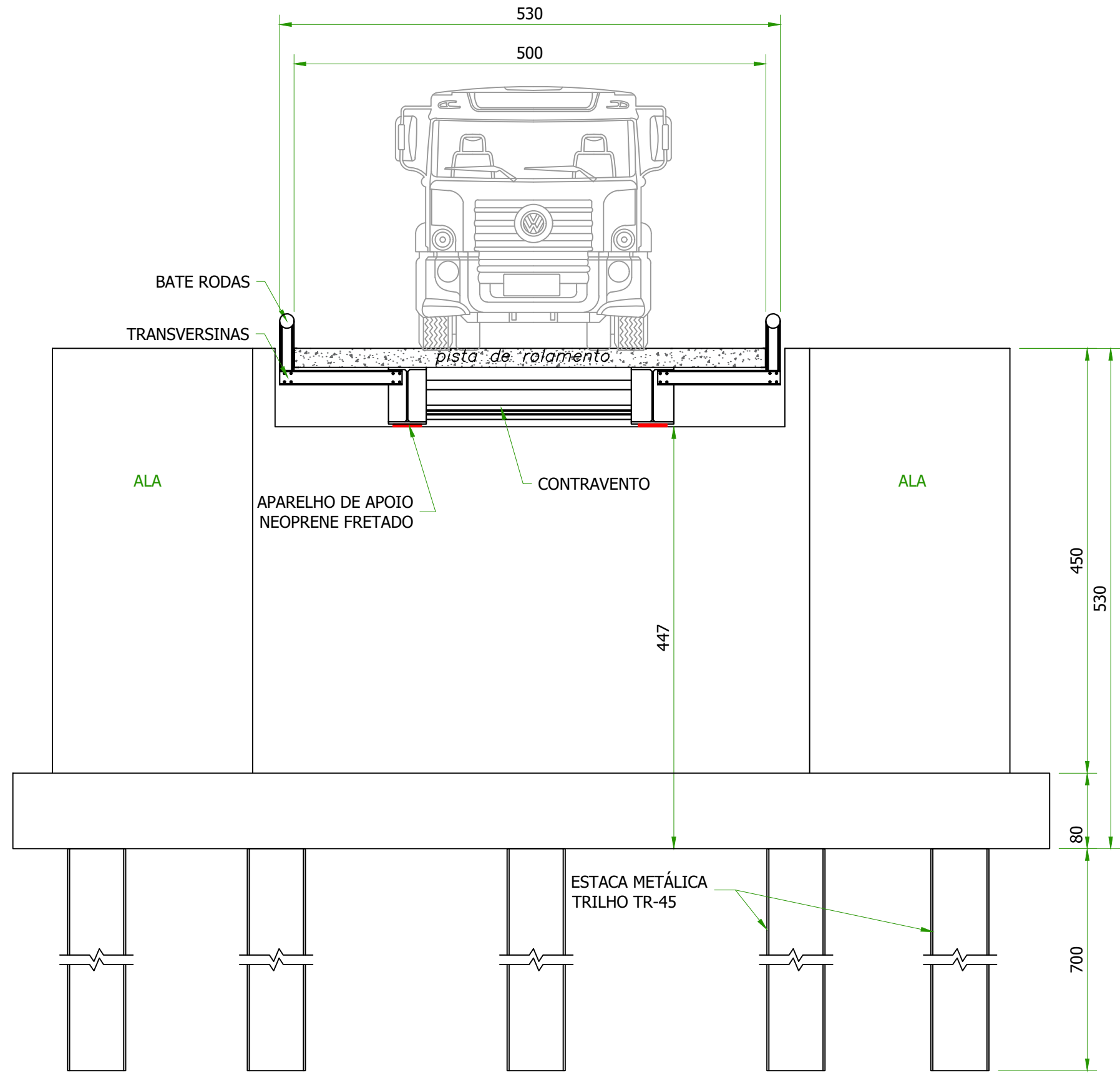
SEÇÃO TRANSVERSAL ESCALA 1:50
