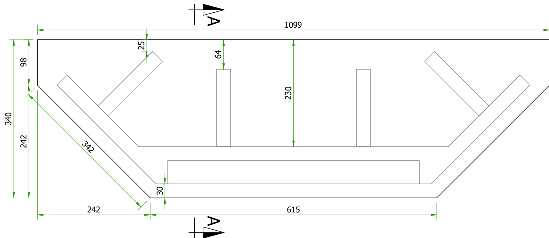
PLANTA BAIXA DO BLOCO ESCALA 1:50
