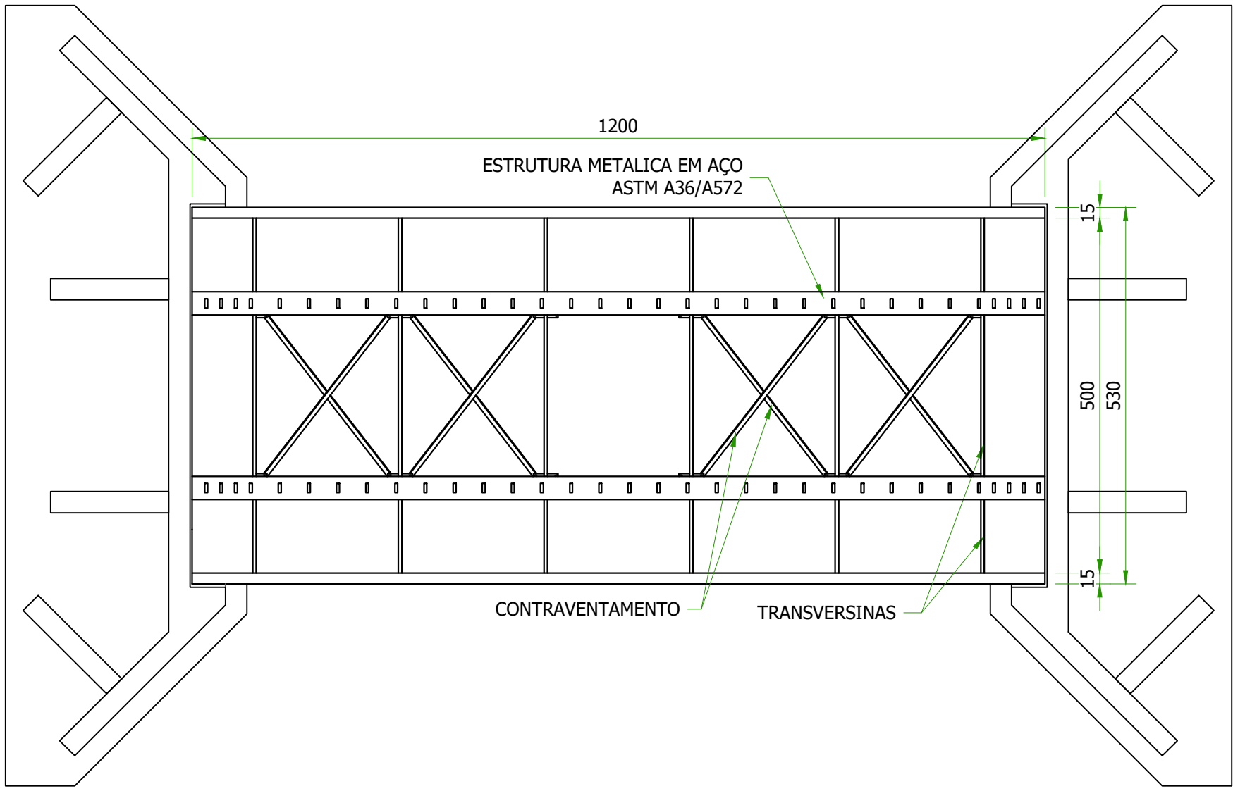
PLANTA DA ESTRUTURA METALICA ESCALA 1:75
