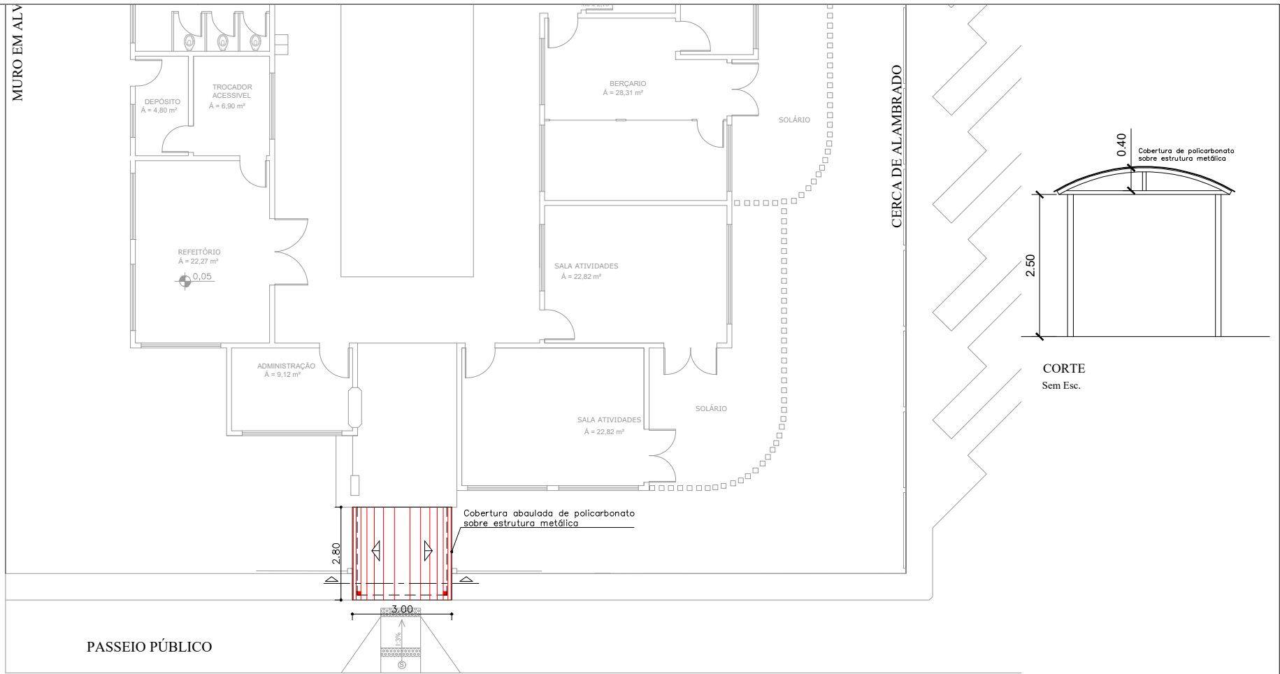
PLANTA BAIXA e COBERTURA Sem Esc.
