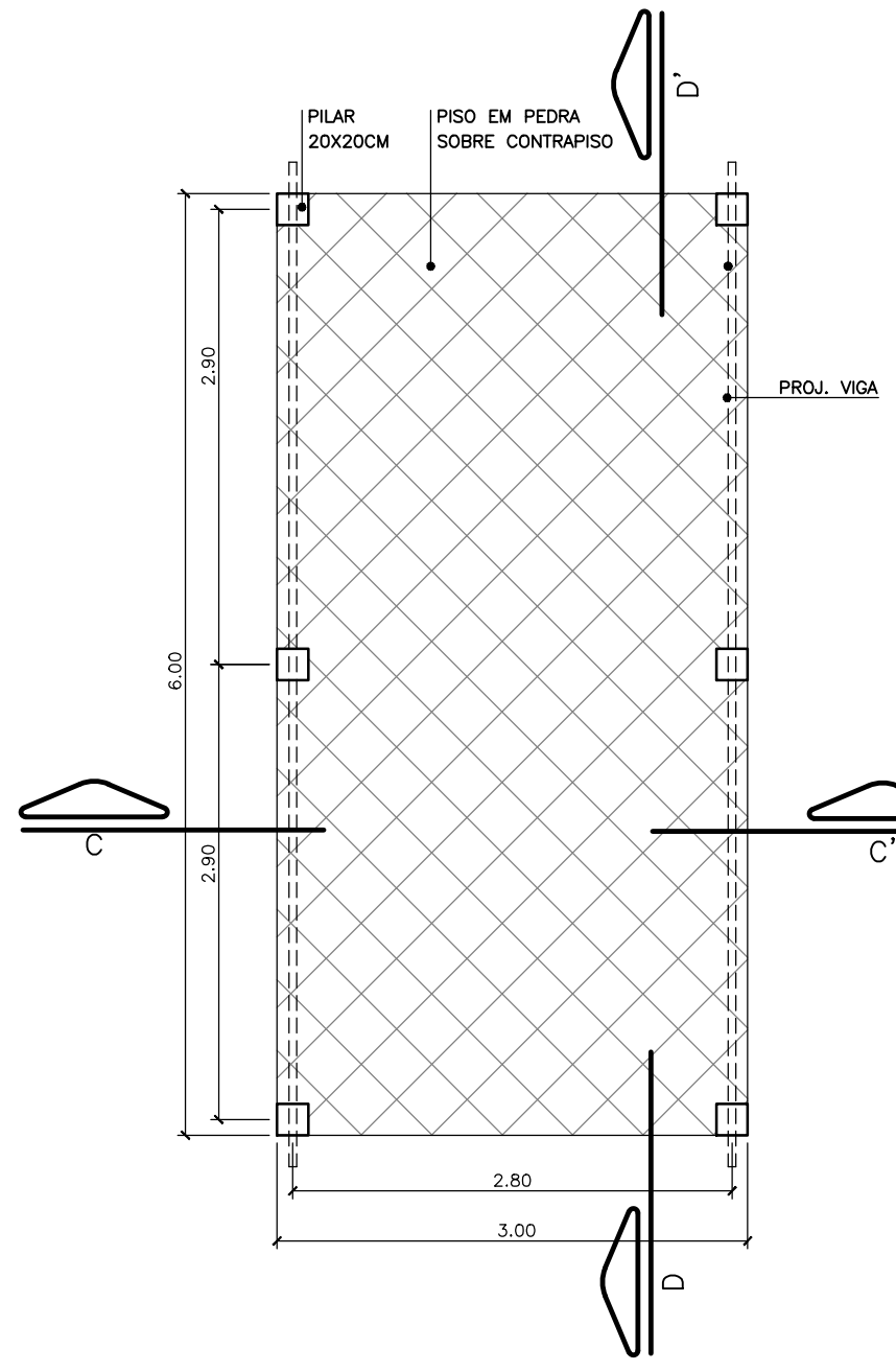
PLANTA DE PISO DO PERGOLADO ESC. 1:50
