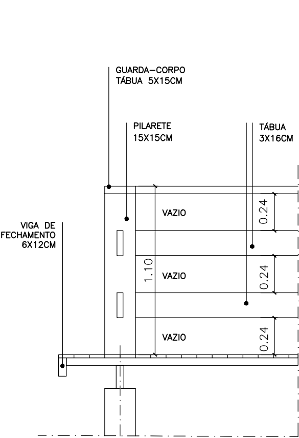
DET. 01 GUARDA-CORPO ESC. 1:25
