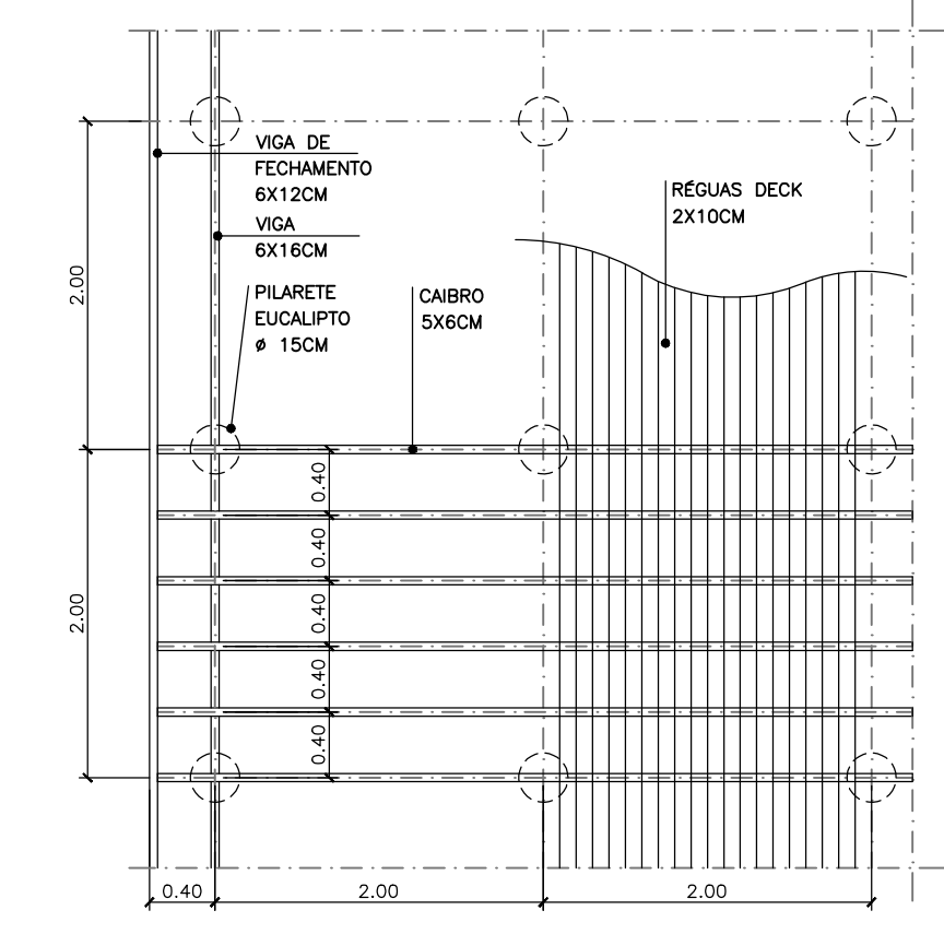
ESTRUTURA DO DECK ESC. 1:50
