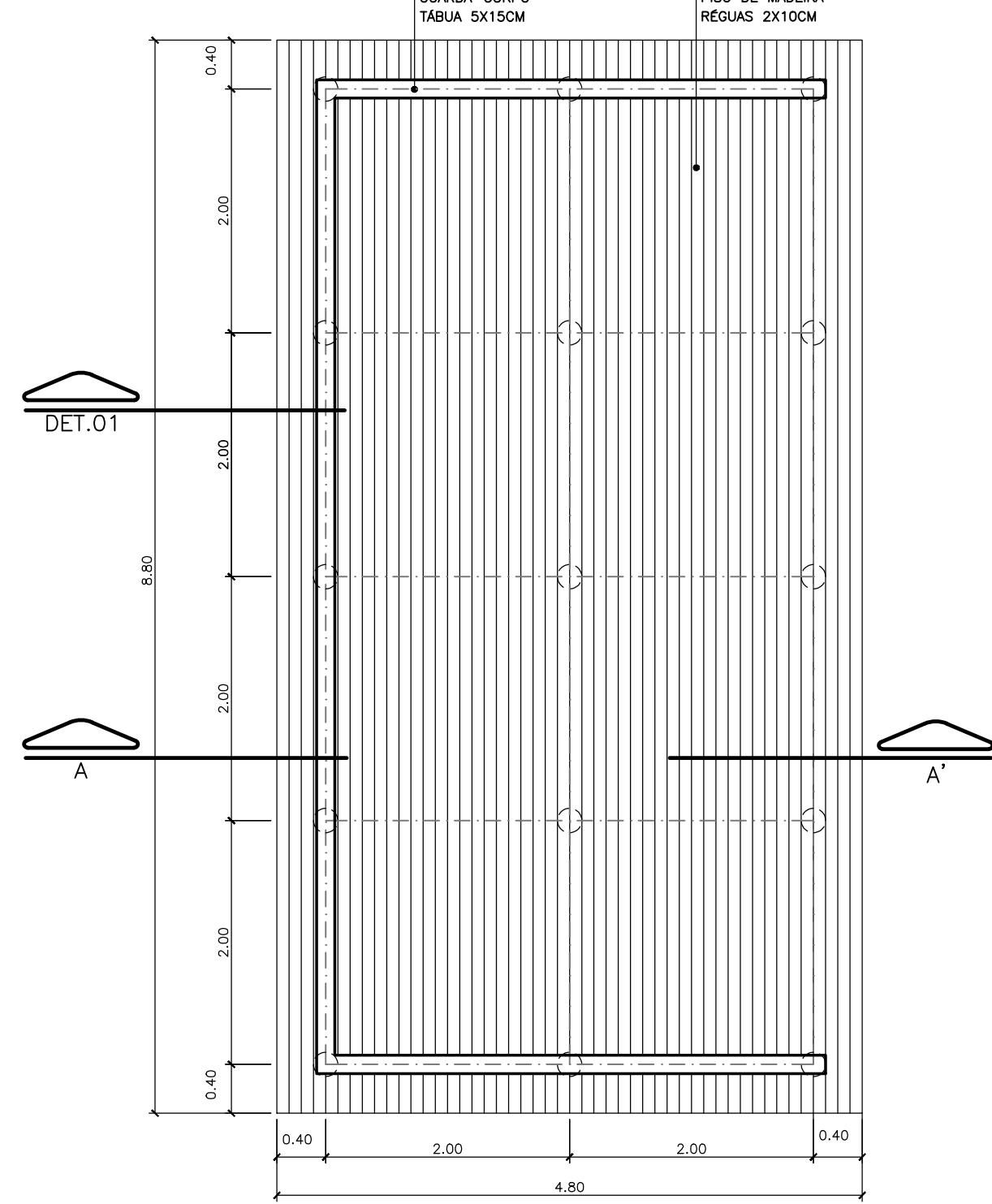
PLANTA DO DECK ESC. 1:50
