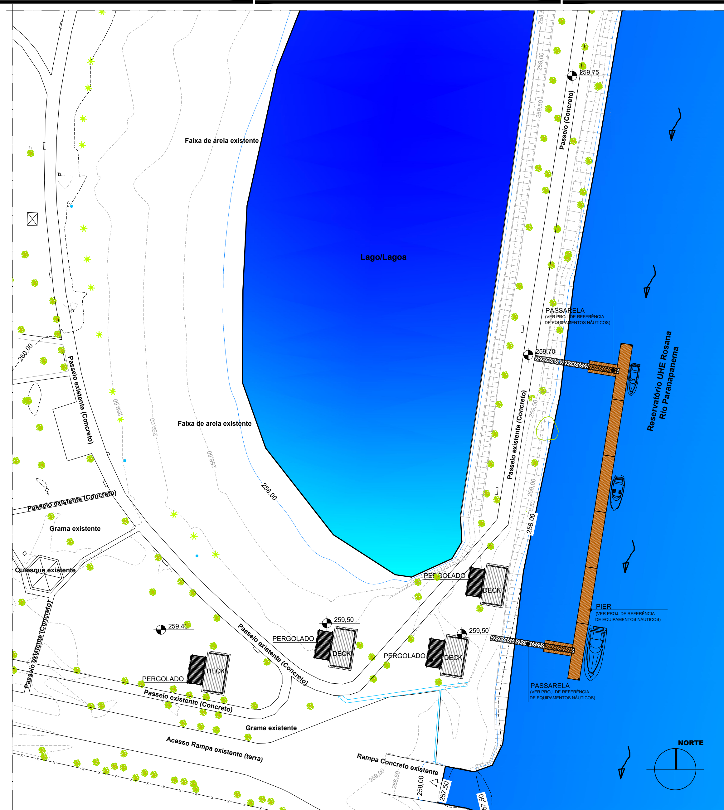
IMPLANTAÇÃO GERAL ESC. 1: 500
