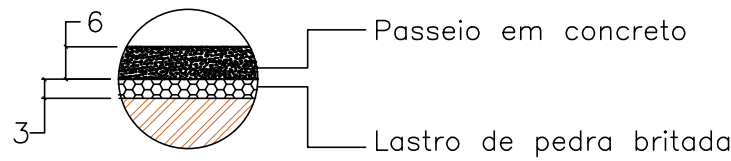
DETALHE PASSEIO/CALÇADA EXTERNA S/ Escala
