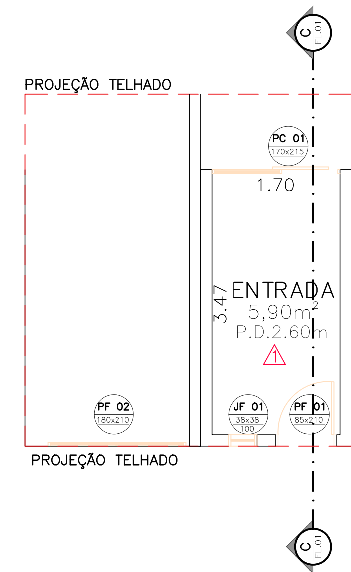
PLANTA BAIXA – ENTRADA GINÁSIO ESC. 1:50
