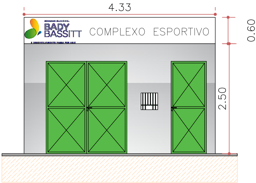
FACHADA ENTRADA ESC. 1:50
