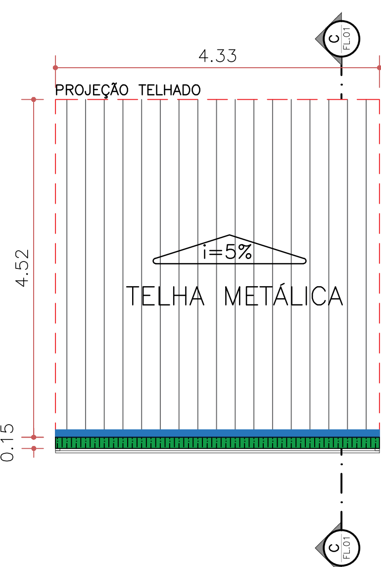
PLANTA COBERTURA – ENTRADA GINÁSIO ESC. 1:50
