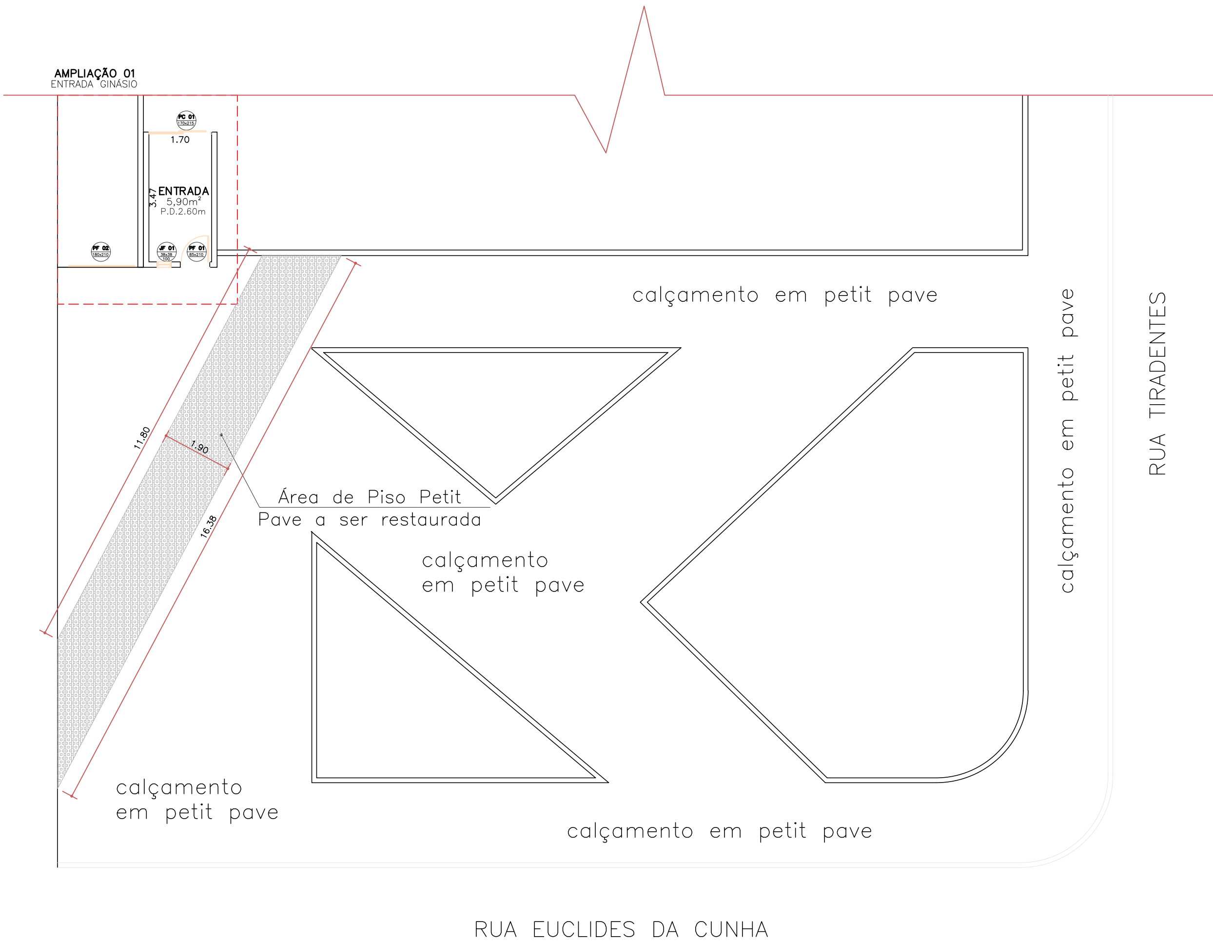
AMPLIAÇÃO 01 – DETALHE CALÇAMENTO EXTERNO ESC. 1:100
