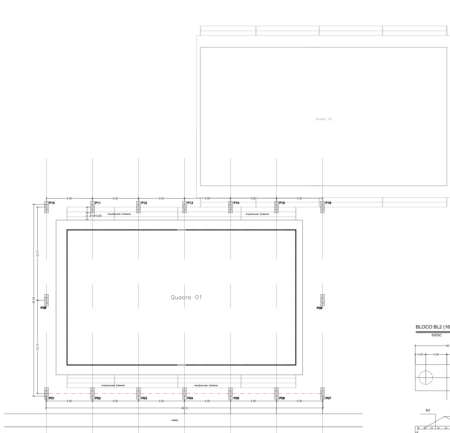
PLANTA-LOCAÇÃO DOS PILARES E BLOCOS ESC. 1:100
