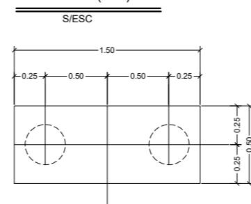
BLOCO BL2 (16X)
