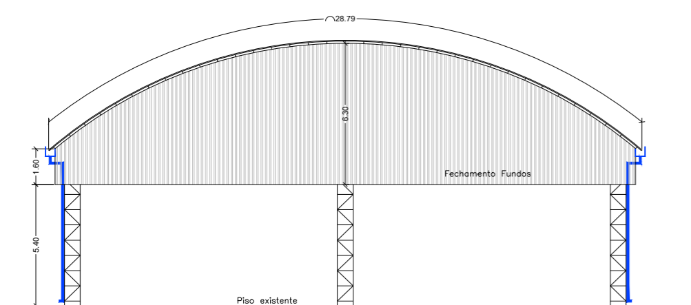
VISTA - FUNDOS ESC. 1:100
