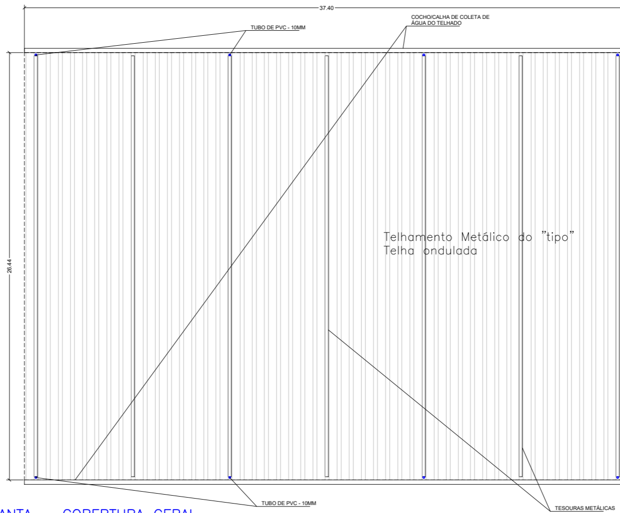
PLANTA - COBERTURA GERAL ESC. 1:100
