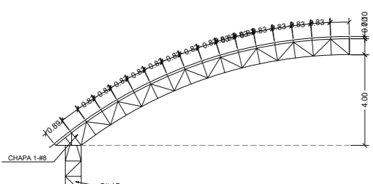
1/2 ARCO (X14) ESC. 1:100
