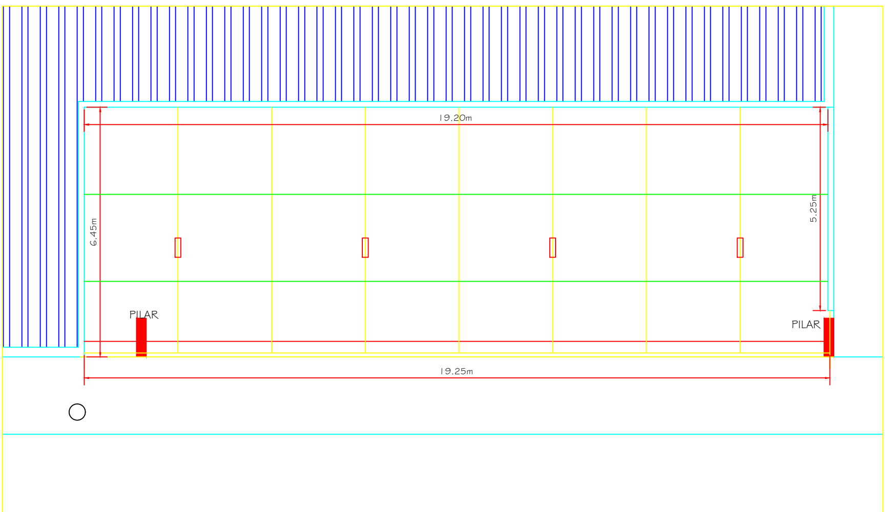
PLANTA DE COBERTURA ESC.: 1/100
