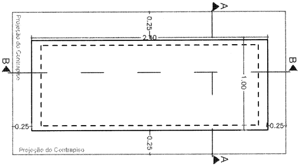
PLANTA S/ESCALA
