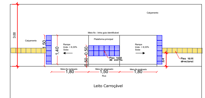
Detalhe 2 - Rampa acessível
