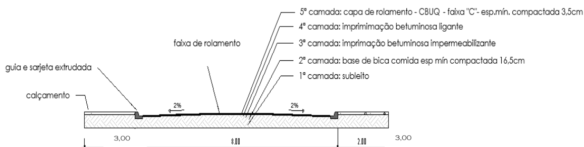
Figura 1: Seção Transversal Tipo da Pavimento Asfáltico
