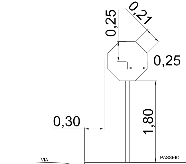
DETALHE 02 DETALHE PARA LOCAÇÃO DE PLACAS Área de Placa de 0,25m²
