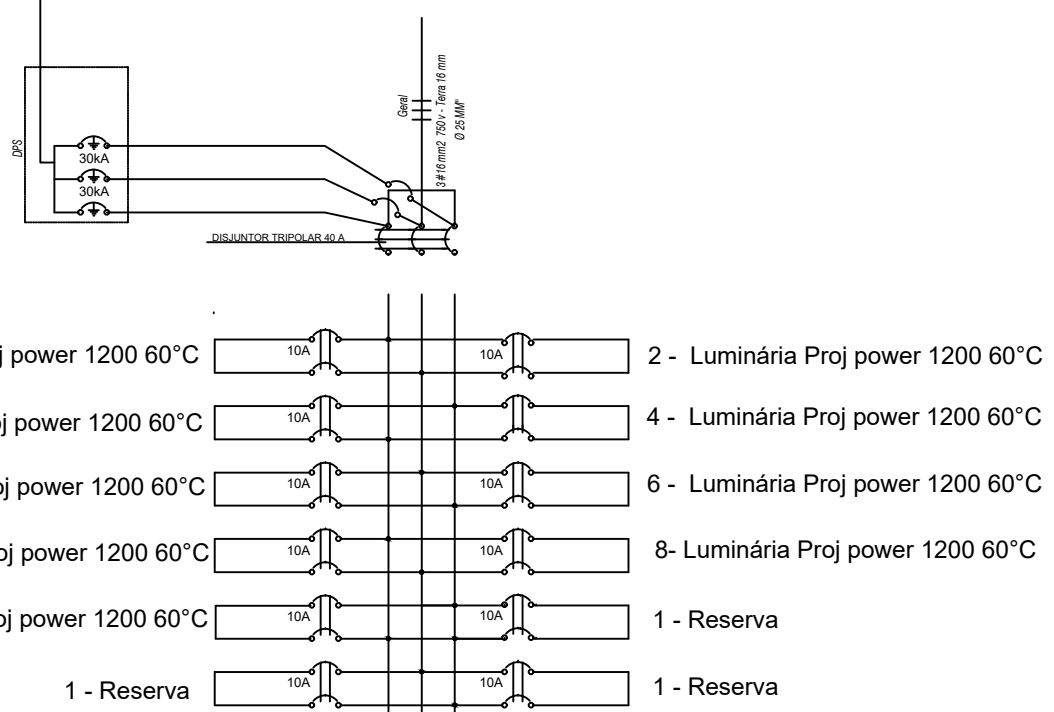
QUADRO DE DISTRIBUIÇÃO 24 DISJUNTORES DIM
