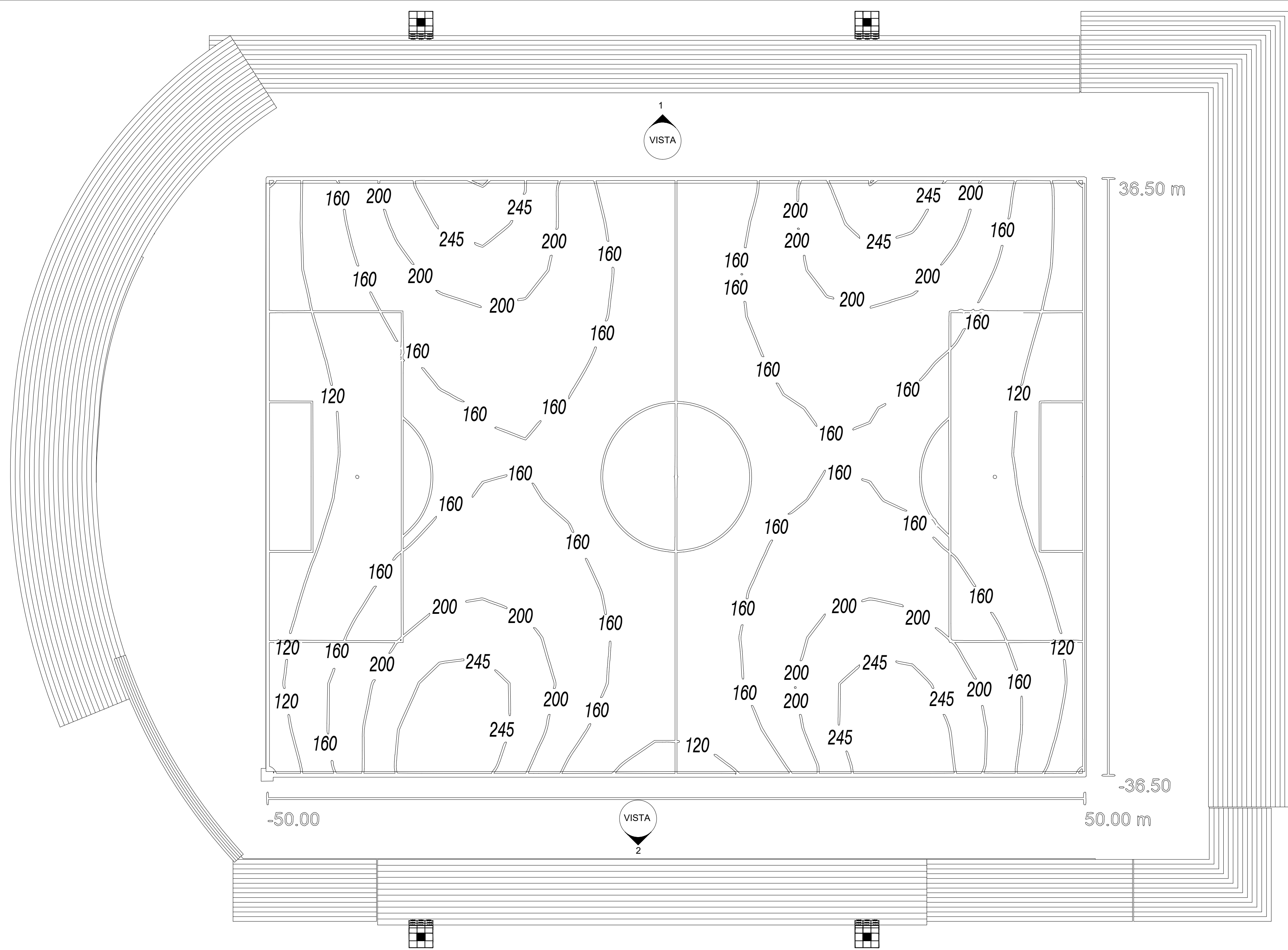
PLANTA VISTA SUPERIOR ESTÁDIO ESC 1:300
