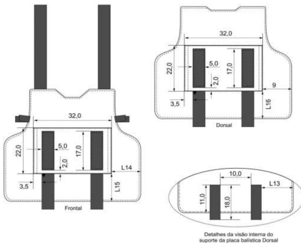
Figura 12 – Vista do velcro do forro
