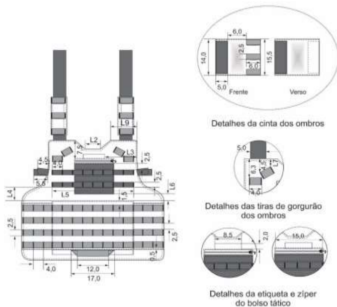
Figura 4 – Detalhes da frente - em centímetros
