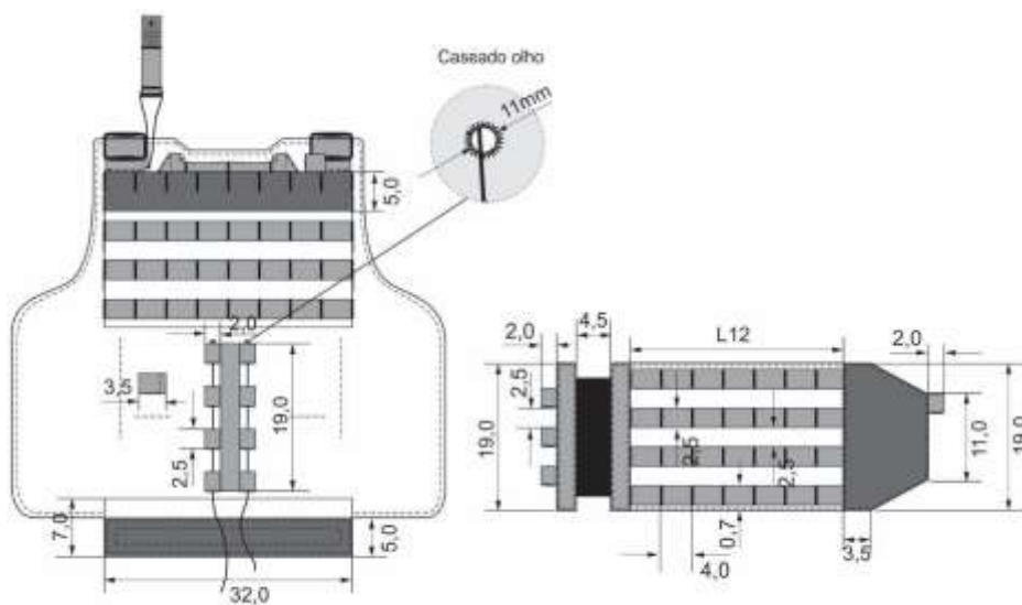
Figura 9 – Detalhes do sistema de soltura rápida do painel lateral – em centímetros
