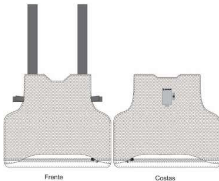
Figura 12 – Vista do velcro do forro
