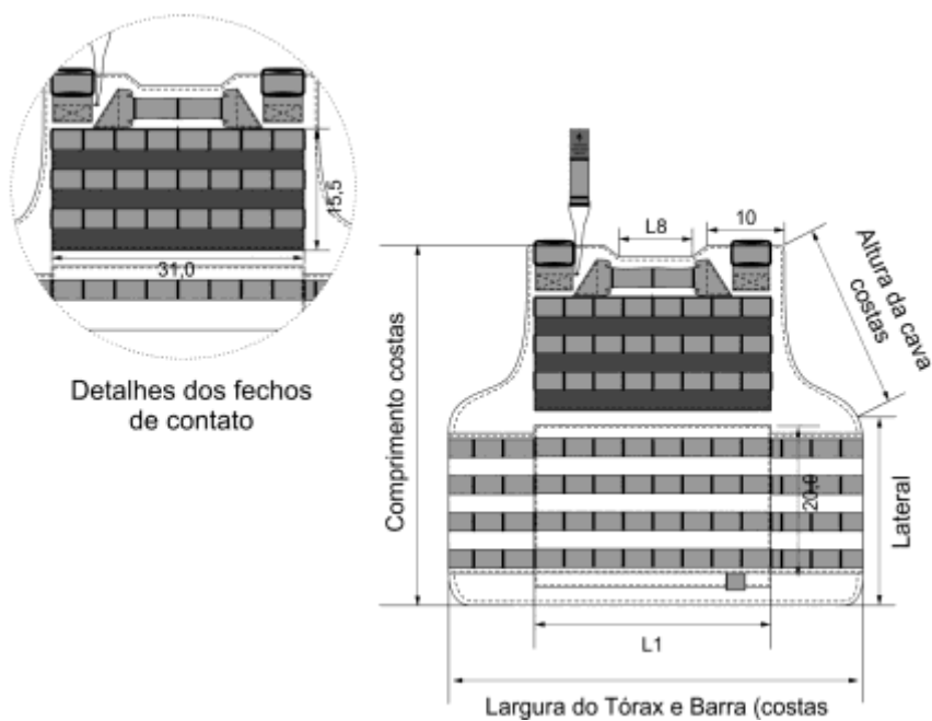
Figura 8 – Detalhes das Costas – em centímetros
