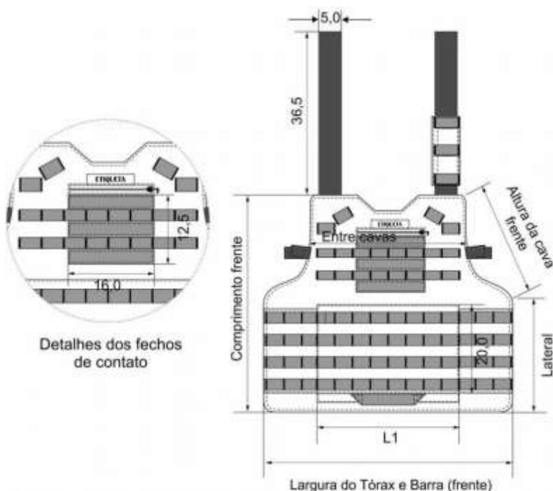
Figura 3 – Medida Base da Frente - em centímetros
