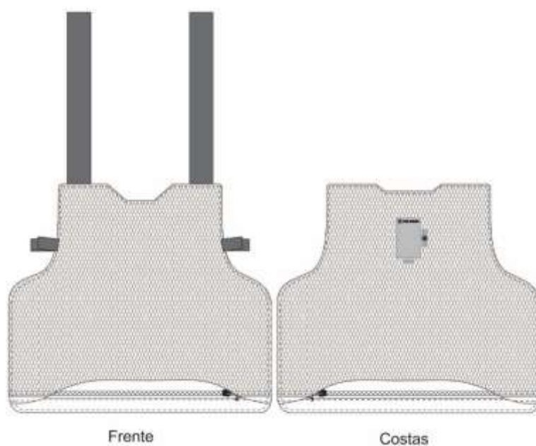
Figura 11 – Vista do forro mesh 3D – em centímetros
