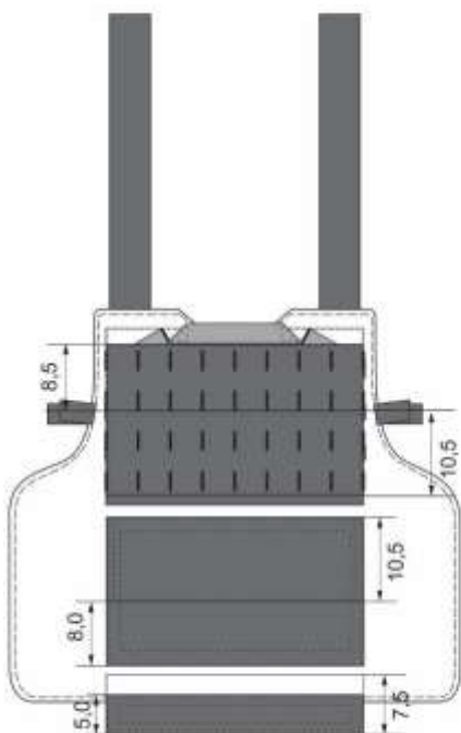
Figura 4 – Detalhes da frente - em centímetros
