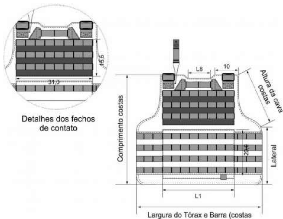
Figura 6 – Vista do painel lateral
