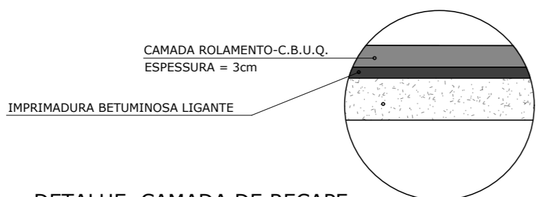
DETALHE CAMADA DE RECAPE S/E
