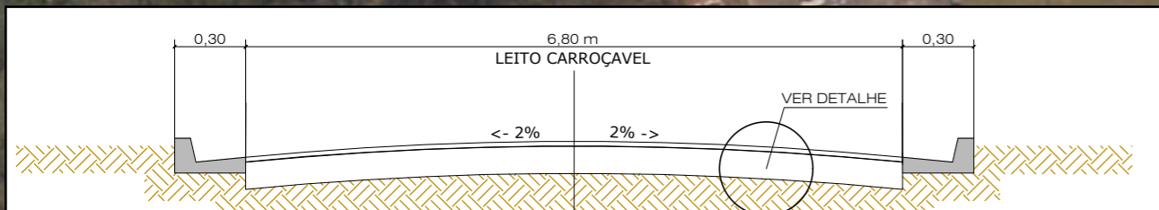
DETALHE - SEÇÃO TRANSVERSAL - PISTA A RECAPEAR S/E
