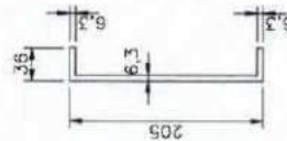
DETALHE CHAPA 1 (mm) ESC: 1:5
