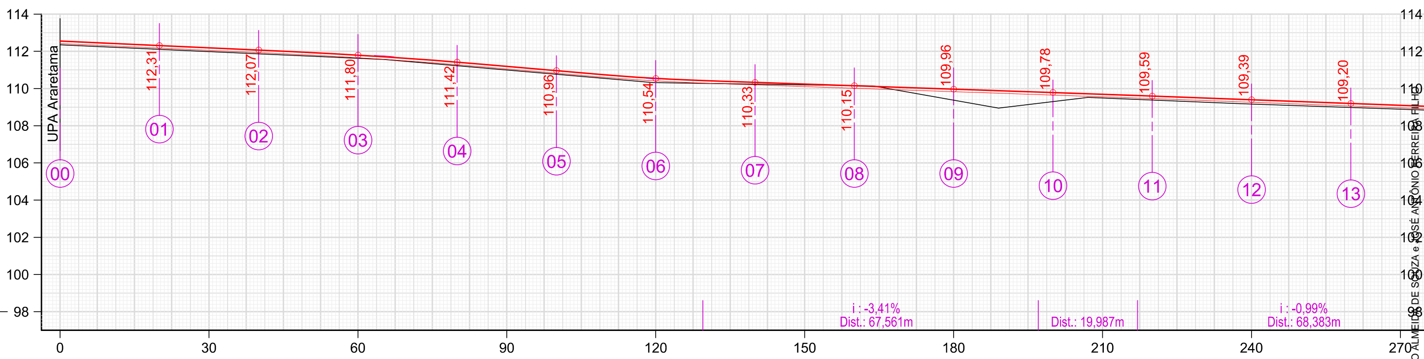
Perfil Longitudinal
