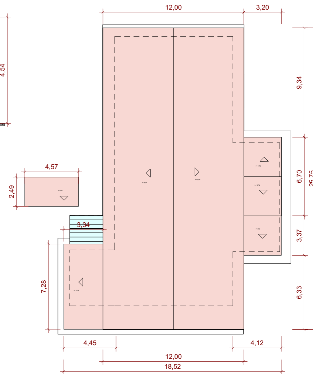
1 COBERTURA 1 : 200
