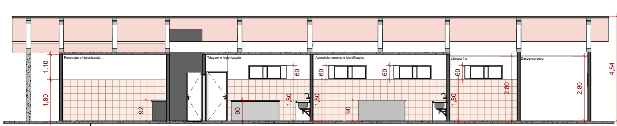
2 CORTE C 1 : 100
