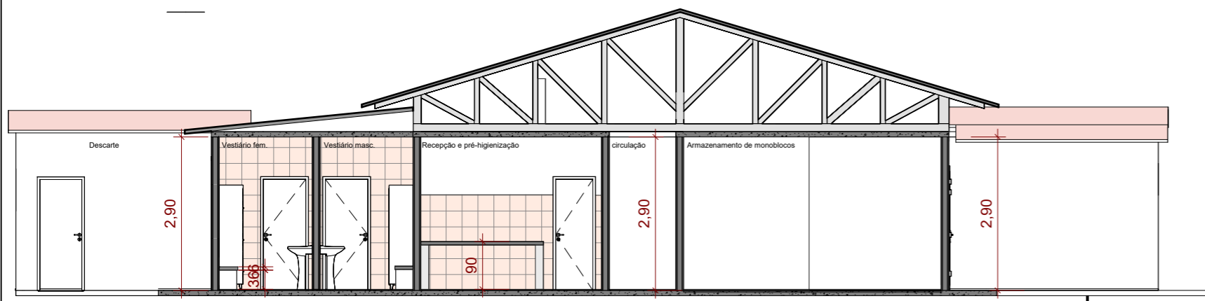
4 CORTE A 1 : 100
