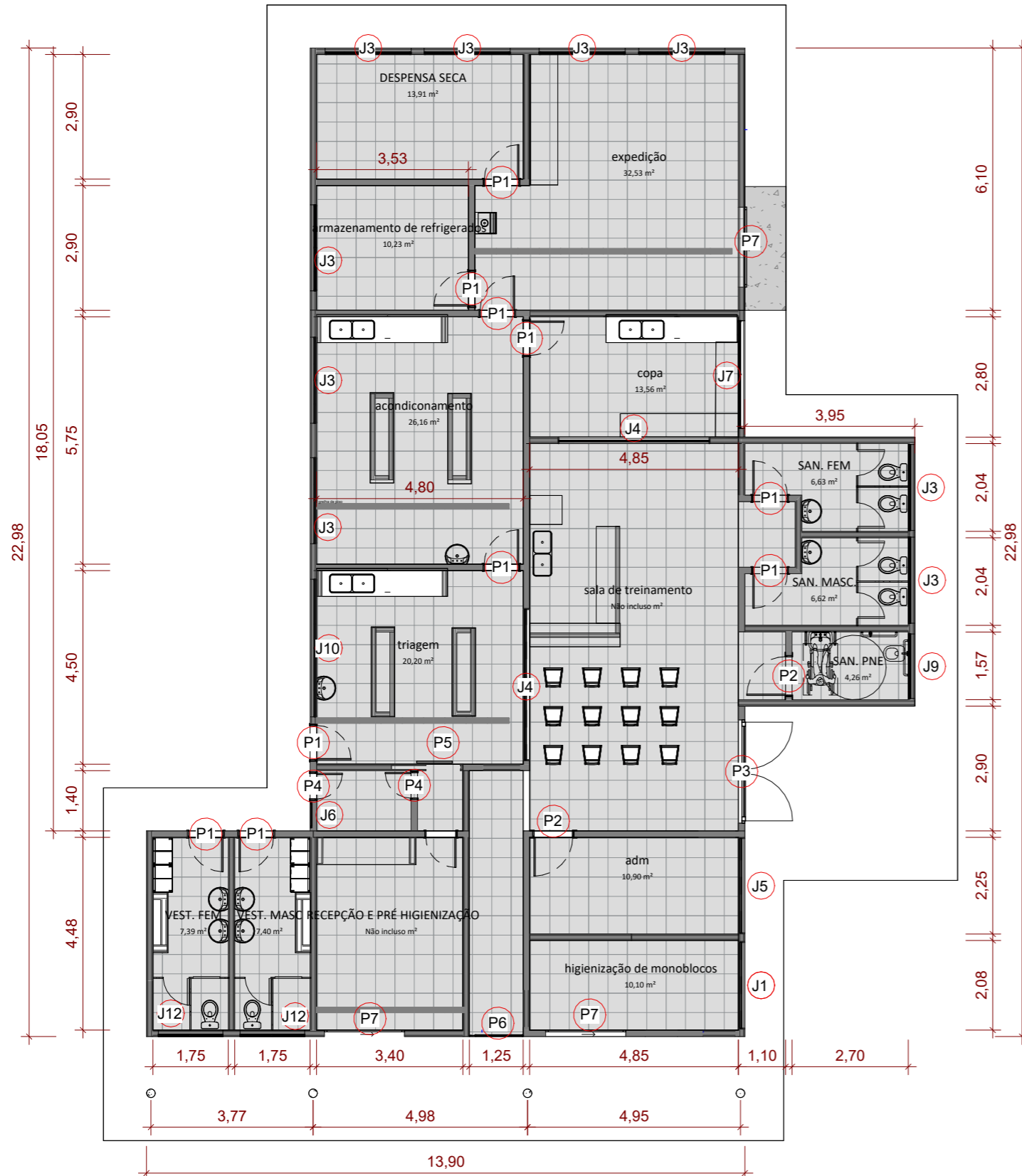
1 IMPLANTAÇÃO 1 : 125
