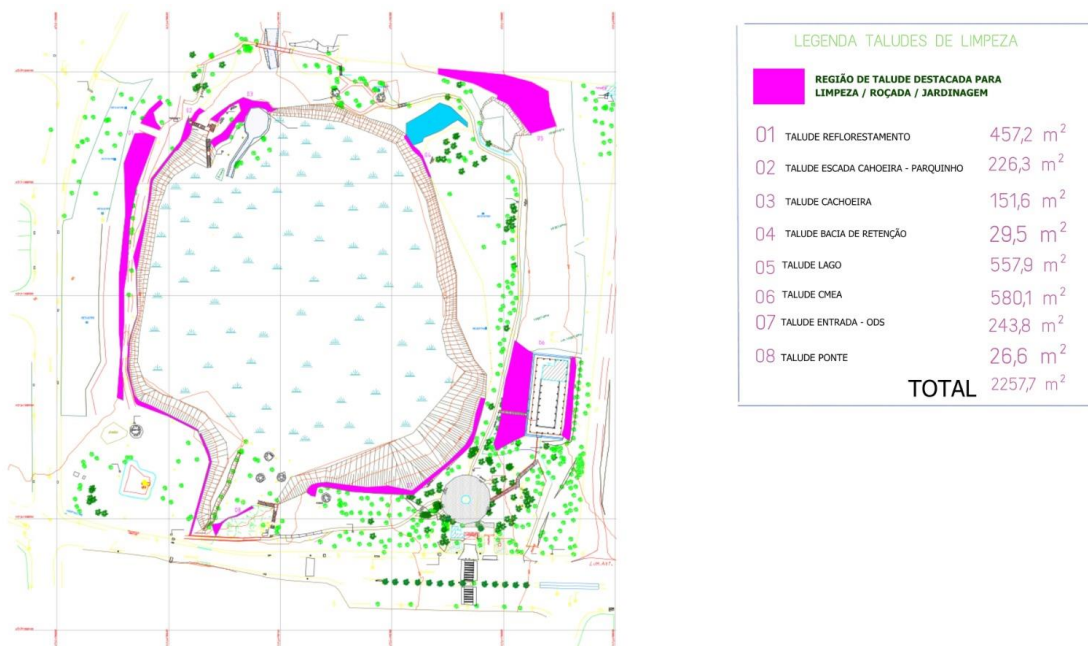
Imagem 2: Esquema de caracterização dos taludes no Parque do Basalto
