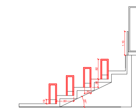
DETALHES CORTE CC ESCALA 1/400
