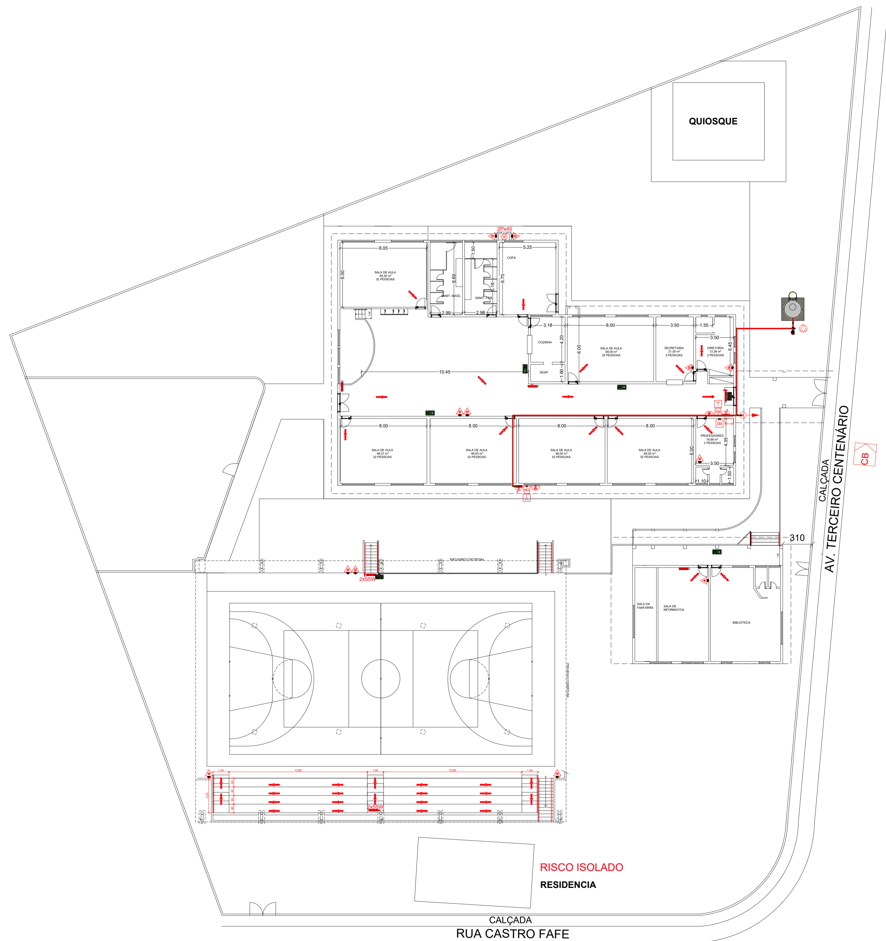
1 : 200 – Planta baixa
