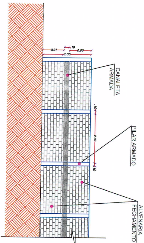
DET. MURO SEM ESCALA
