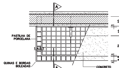
DETALHE 1 Esc.: 1:20
