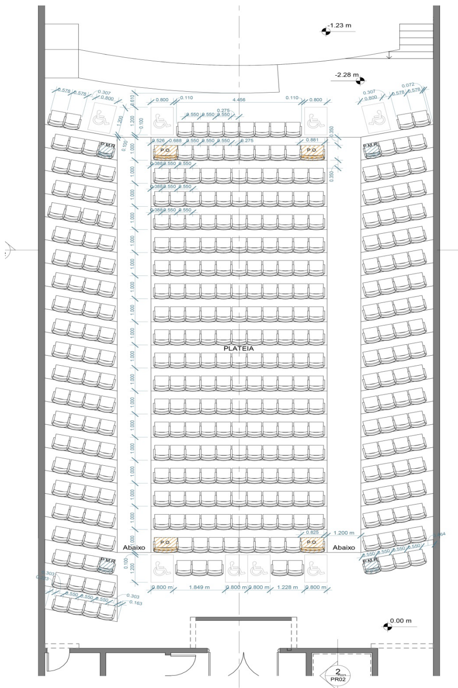
PLANTA BAIXA PAV. PLATEIA - INDICAÇÕES POLTRONAS
