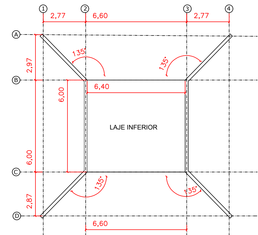
LOCAÇÃO ESC: 1:100
