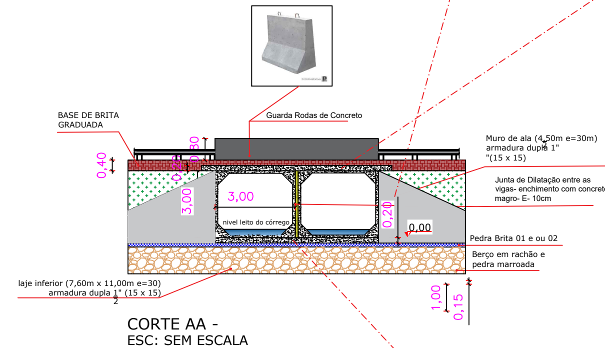
CORTE AA - ESC: SEM ESCALA
