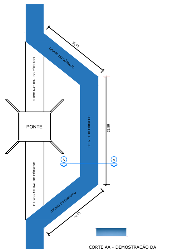
DESVIO TEMPORÁRIO CURSO D'ÁGUA (CORTA RIO) - ITEM 3.1
