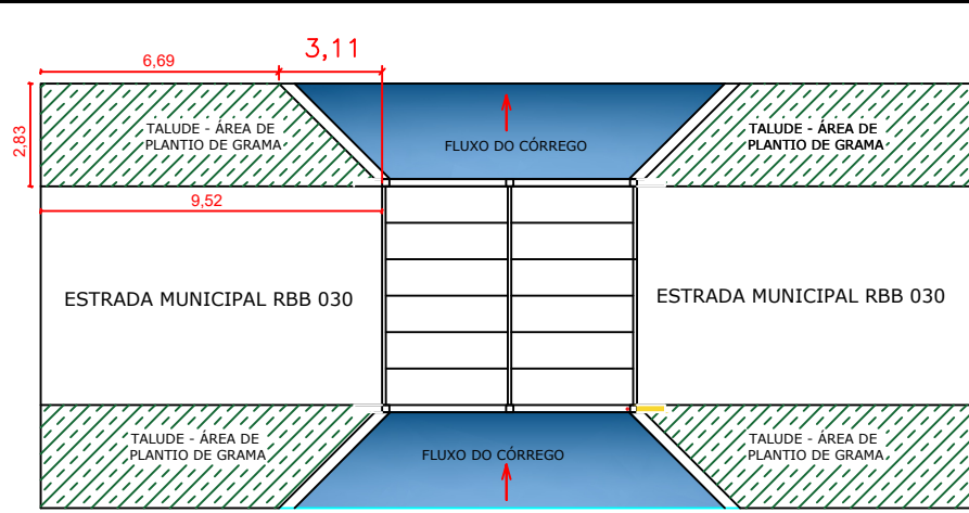
PLANTO DE GRAMA - ITEM 7.1 ESC: 1:100
