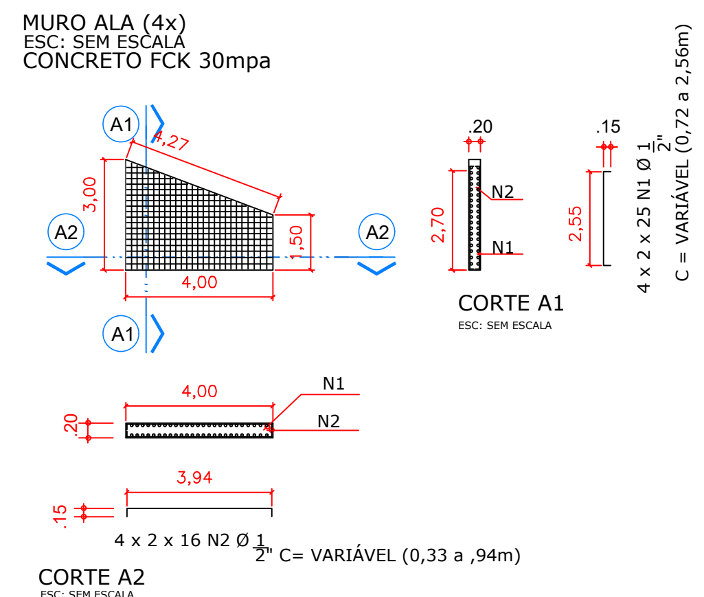
CORTE A1 ESC: SEM ESCALA
