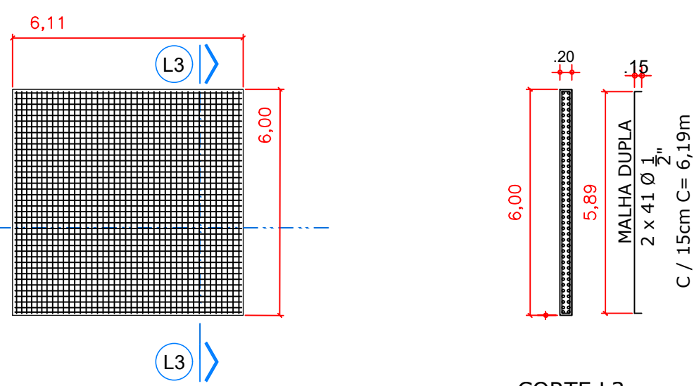
CORTE L4 ESC: 1:100
