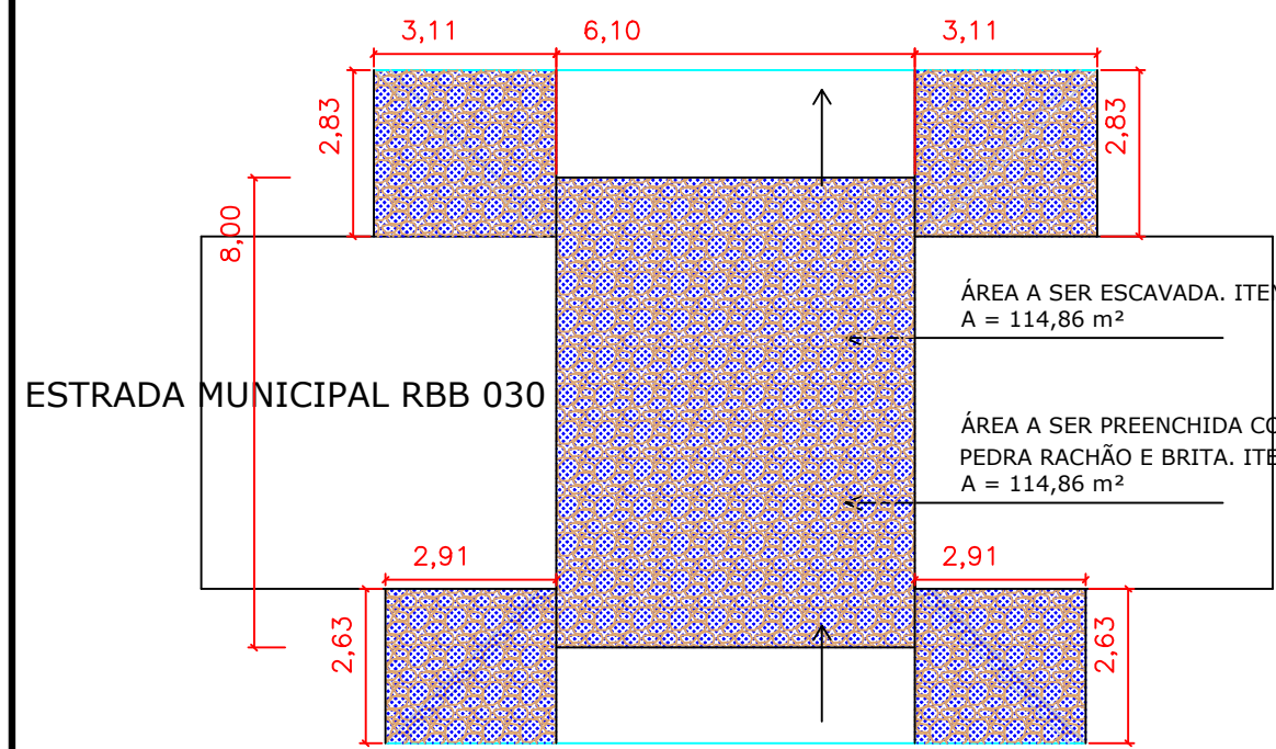
PLANTA DE LOCALIZAÇÃO DA ESCAVAÇÃO DE SOLO MOLE E INSTALAÇÃO DA PEDRA RACHÃO E PEDRA BRITA - Item 3.3, 3.4, 3.5 e 3.6 ESC: 1:100
