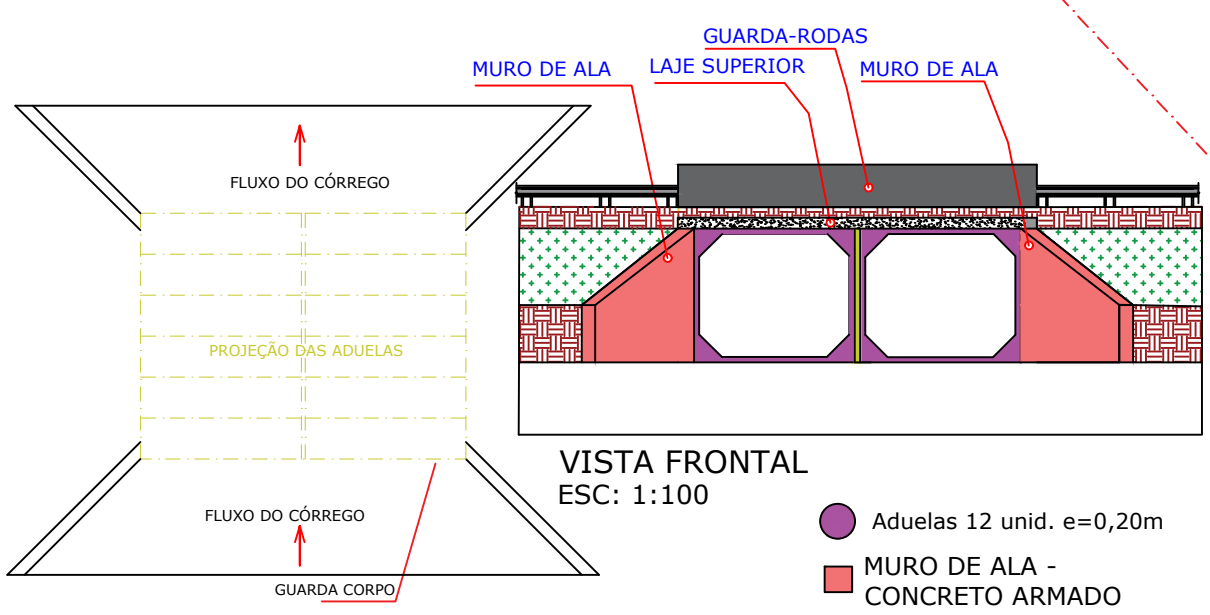
PLANTA BAIXA PROJEÇÃO ADUELAS - Item 3.7 ESC: 1:100
