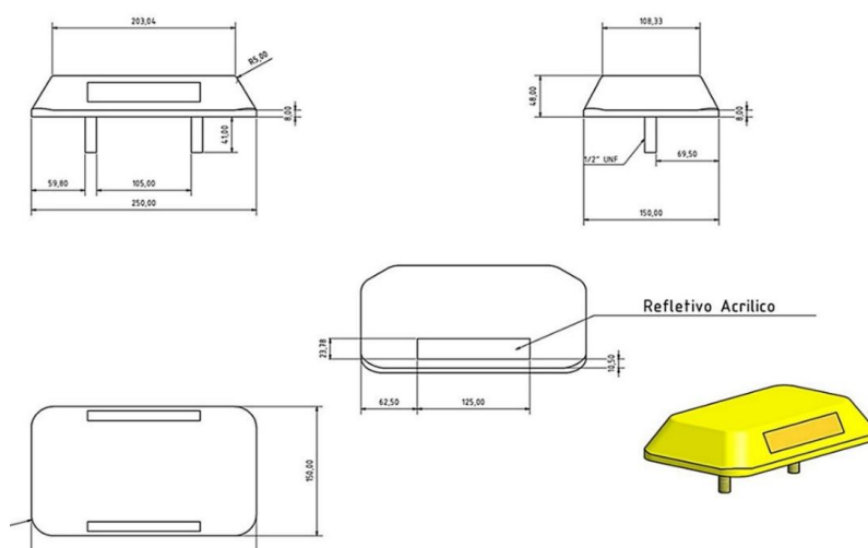
Figura 2: Tachões refletivos para sinalização – Corpo em ABS
