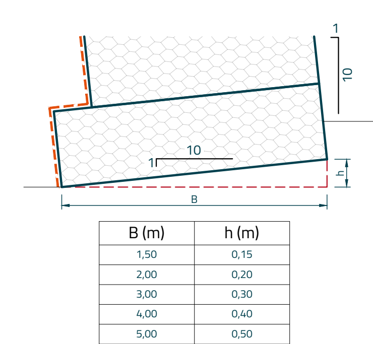
Detalhe de Preparação da Base Sem Escala
