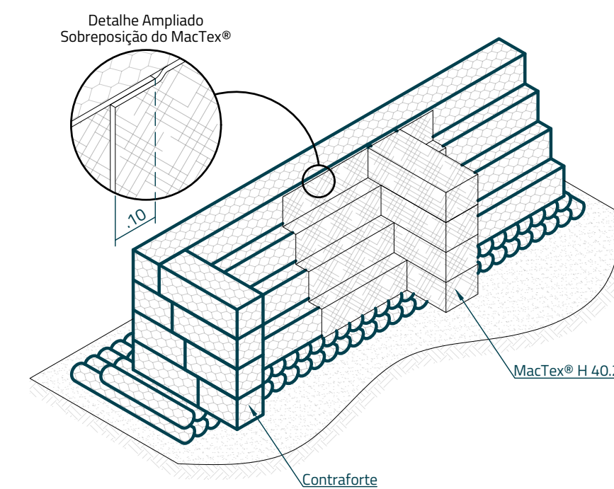
Detalhe em Perspectiva dos contrafortes Sem Escala
