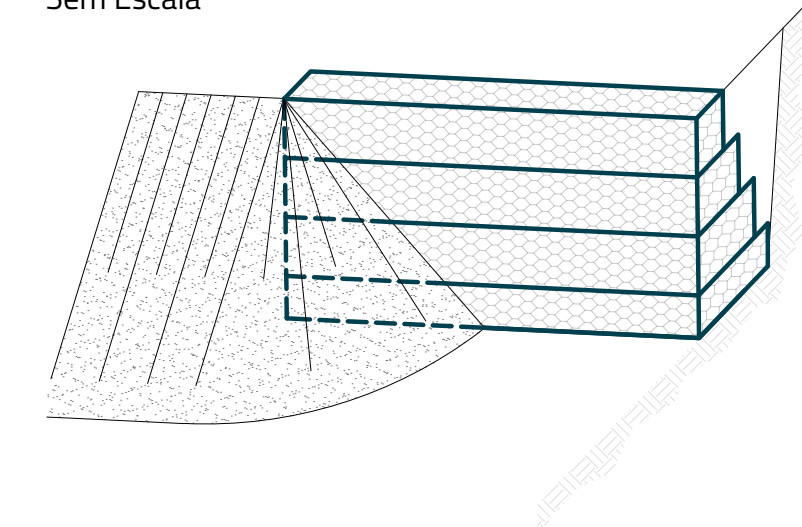
Detalhe do Fechamento Lateral Sem Escala
