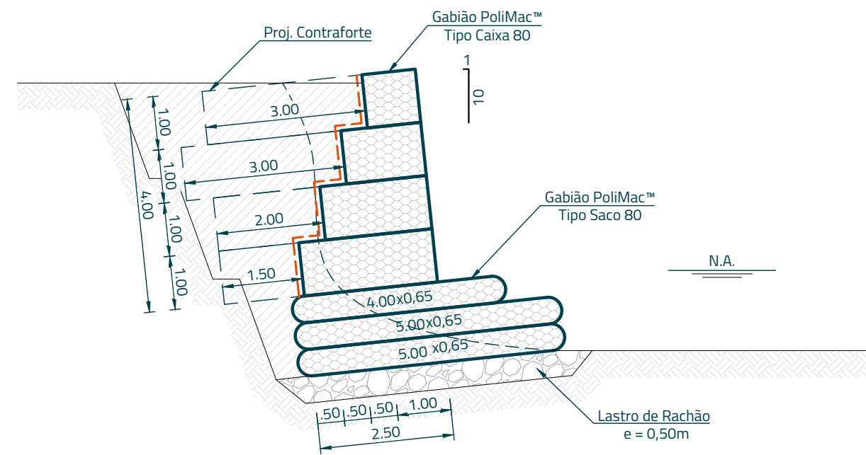
Seção Típica | Extensão: 50.00m | Escala 1:100
