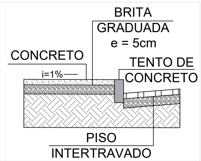
DETALHE 02 - PISOS - CIMENTO/INTERTRAVADO ESC. 1:25
