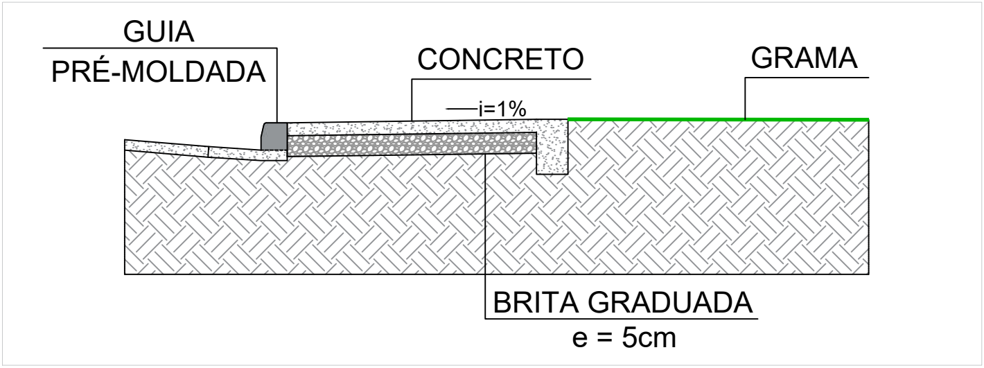
DETALHE 03 - PISOS - CIMENTO/GRAMA ESC. 1:25
