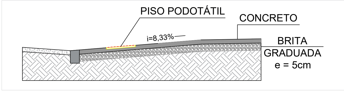
CORTE - RAMPAS ACESSIBILIDADE ESC. 1:25
