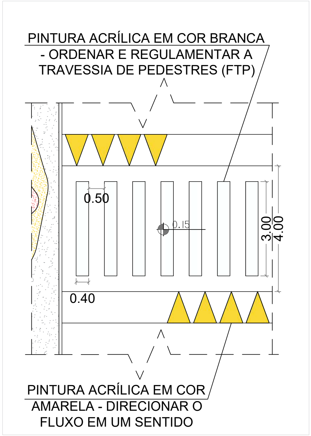
DETALHE - FAIXA ELEVADA ESC. 1:50
