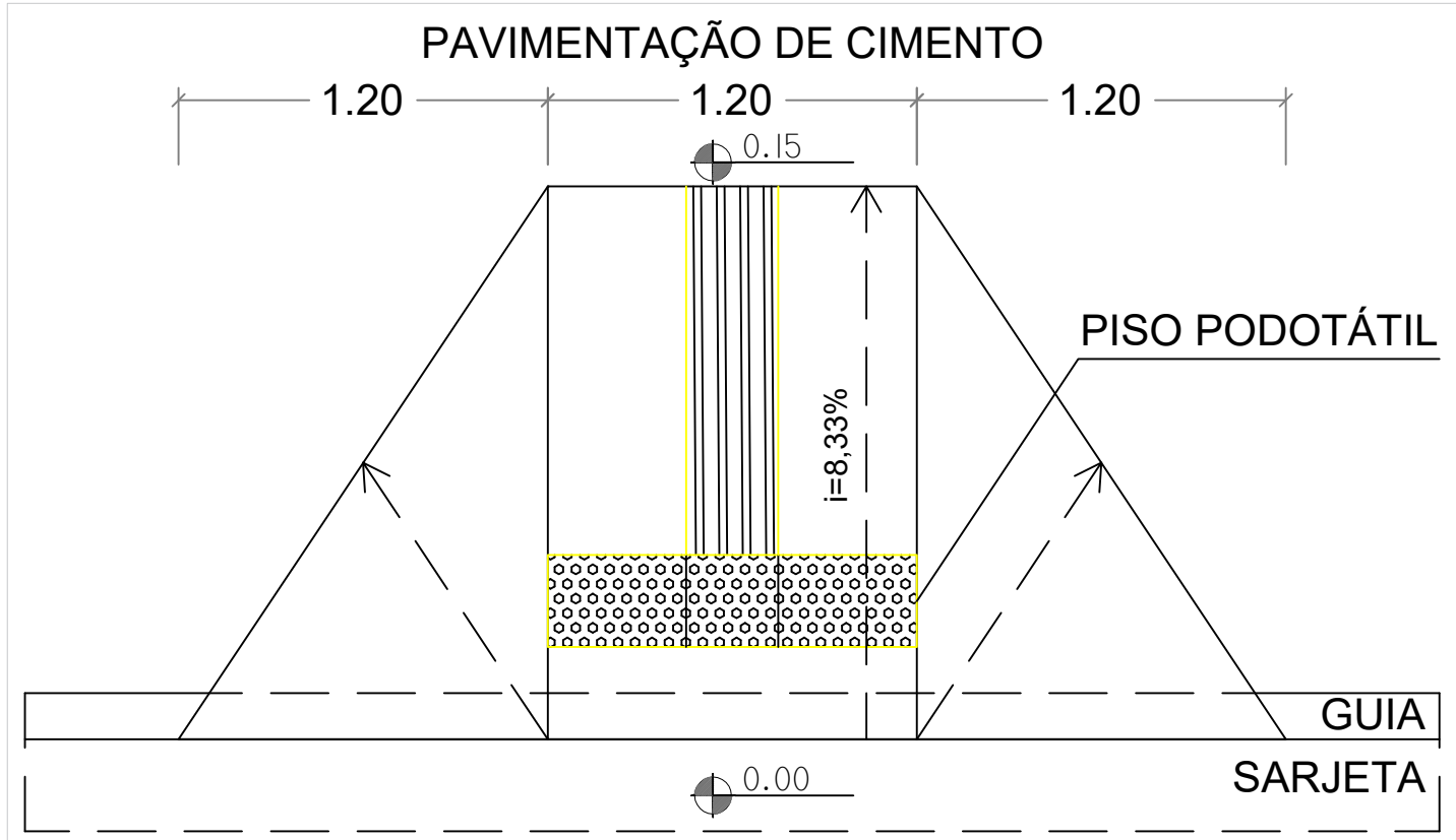
DETALHE - RAMPAS ACESSIBILIDADE ESC. 1:25
