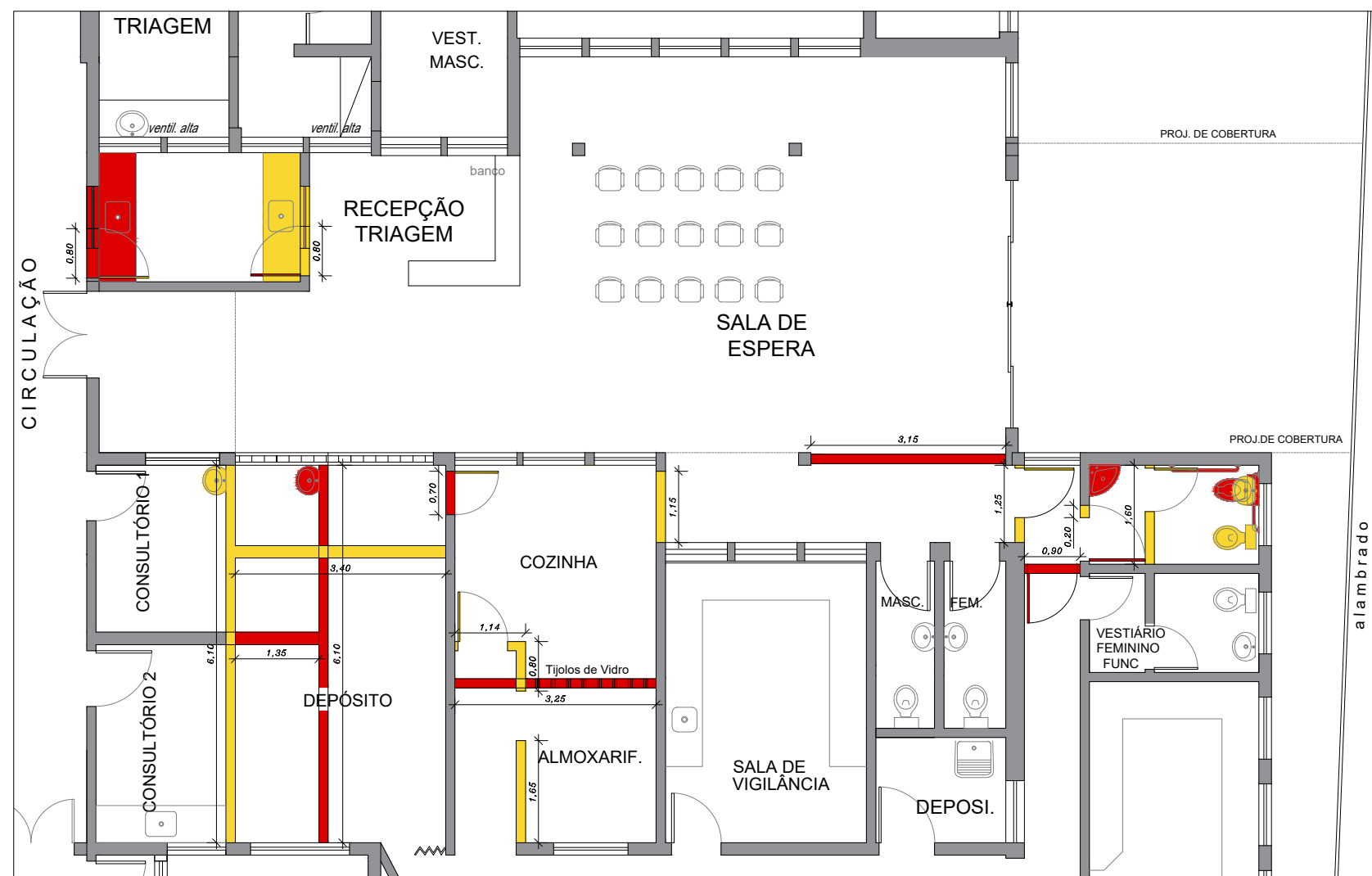
PLANTA DE REFORMA ESCALA 1:100
