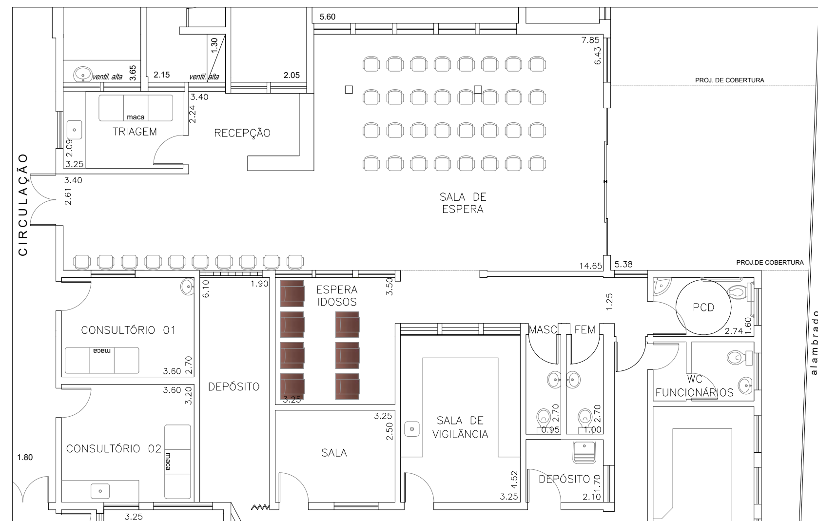
PLANTA DE LAYOUT ESCALA 1:100
