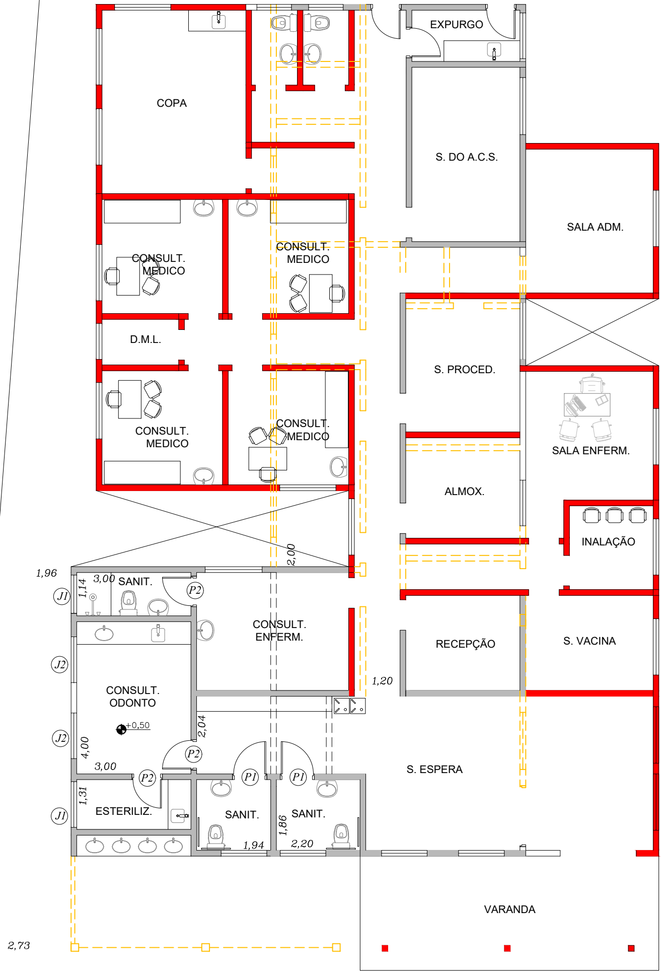
PLANTA DA SITUAÇÃO EXISTENTE ESCALA 1:100
