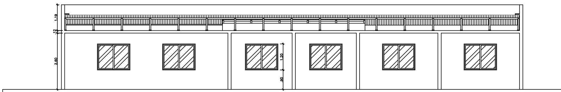
CORTE C-C
