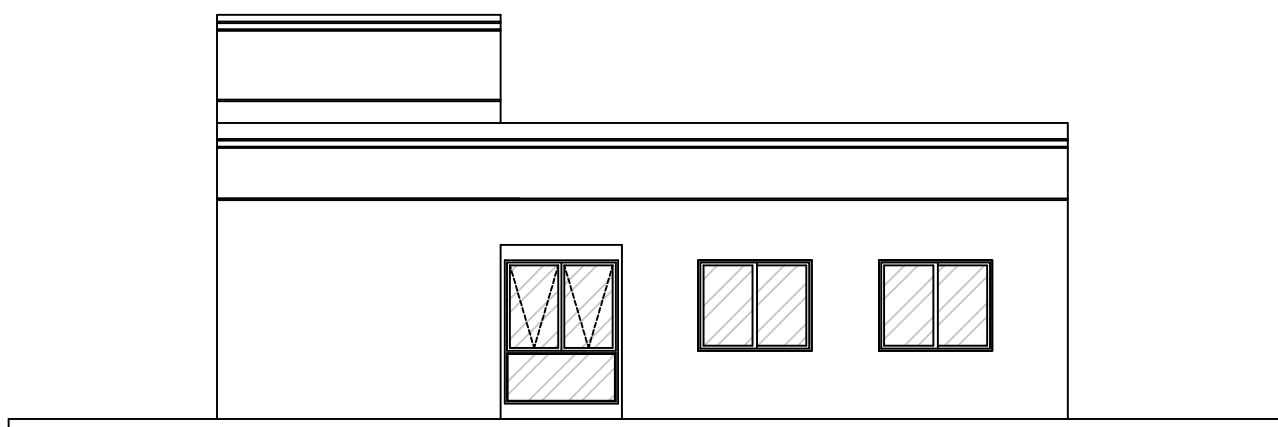
FACHADA POSTERIOR
