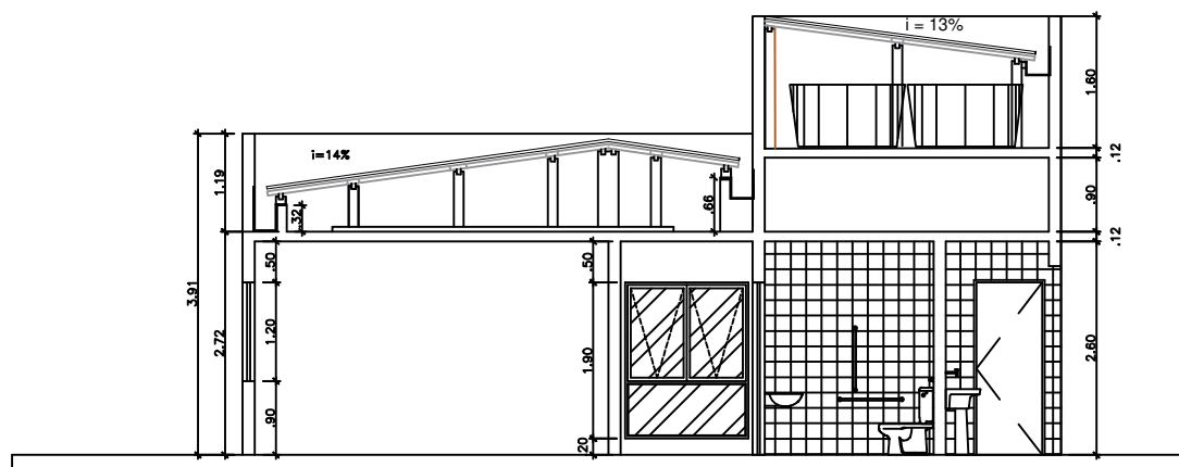
CORTE B-B
