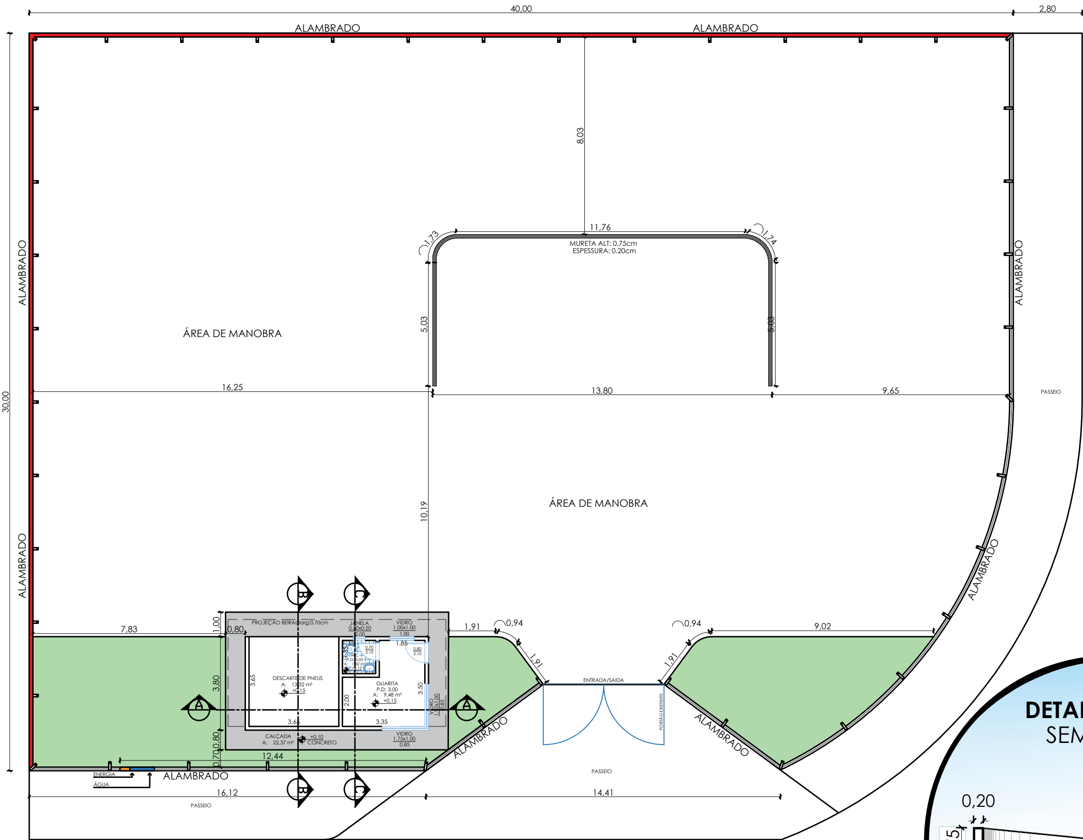
PLANTA BAIXA - ECOPONTO ESC 1/150
