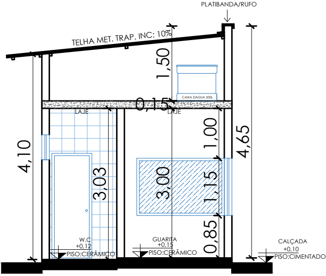
CORTE CC- ECOPONTO ESC 1/75
