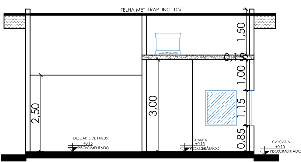
CORTE AA- ECOPONTO ESC 1/75
