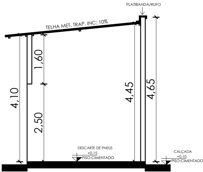
CORTE BB- ECOPONTO ESC 1/75
