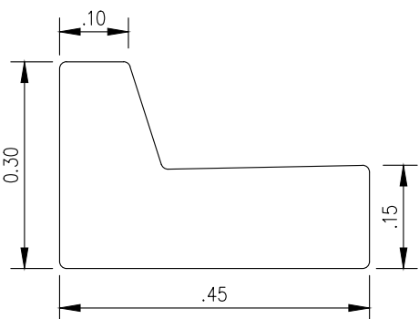
DET. PERFIL GUIA/SARJETA S/ESCALA - MEDIDAS EM (M)
