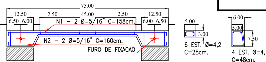
DETALHE DA VIGA 5 ESCALA = 1:10
