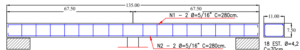
DETALHE DA VIGA 6 ESCALA = 1:20
