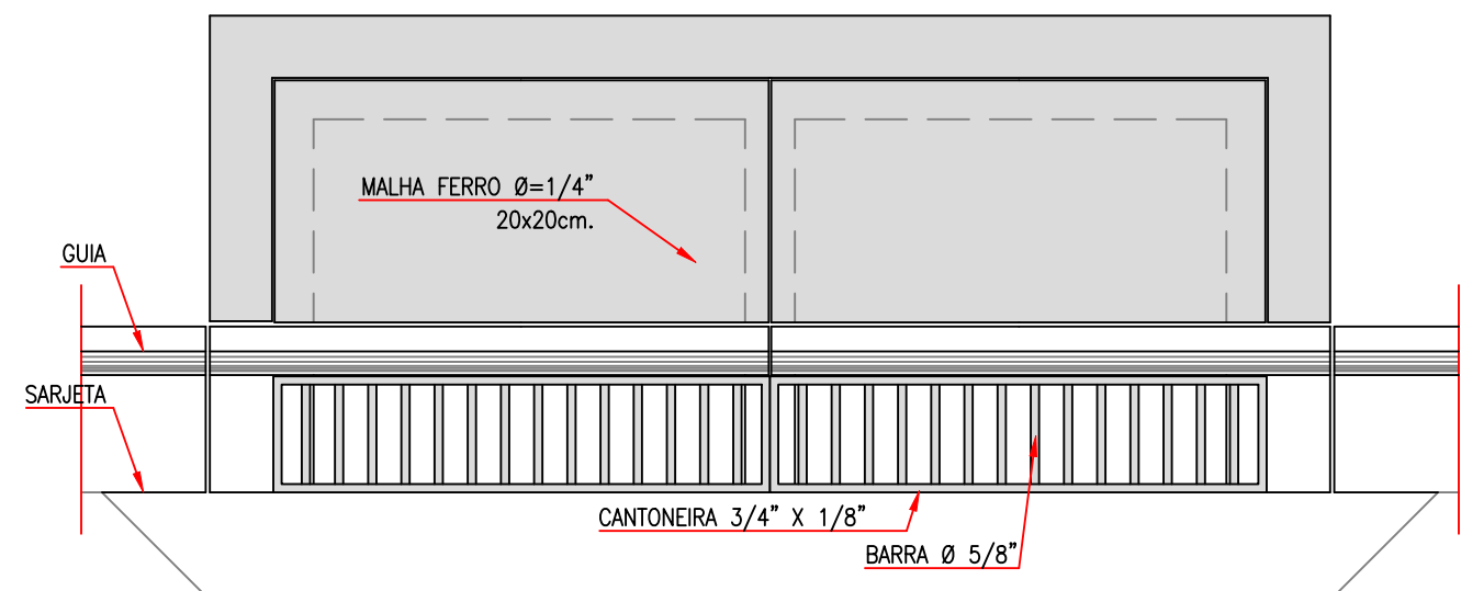
VISTA SUPERIOR ESCALA = 1:20
