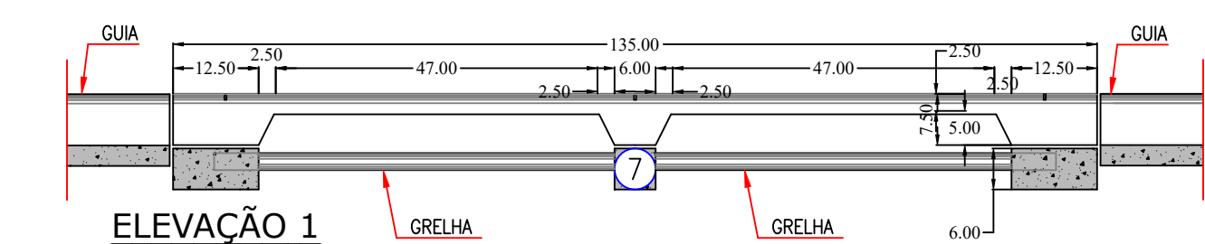
ELEVACÃO 1 ESCALA = 1:20
