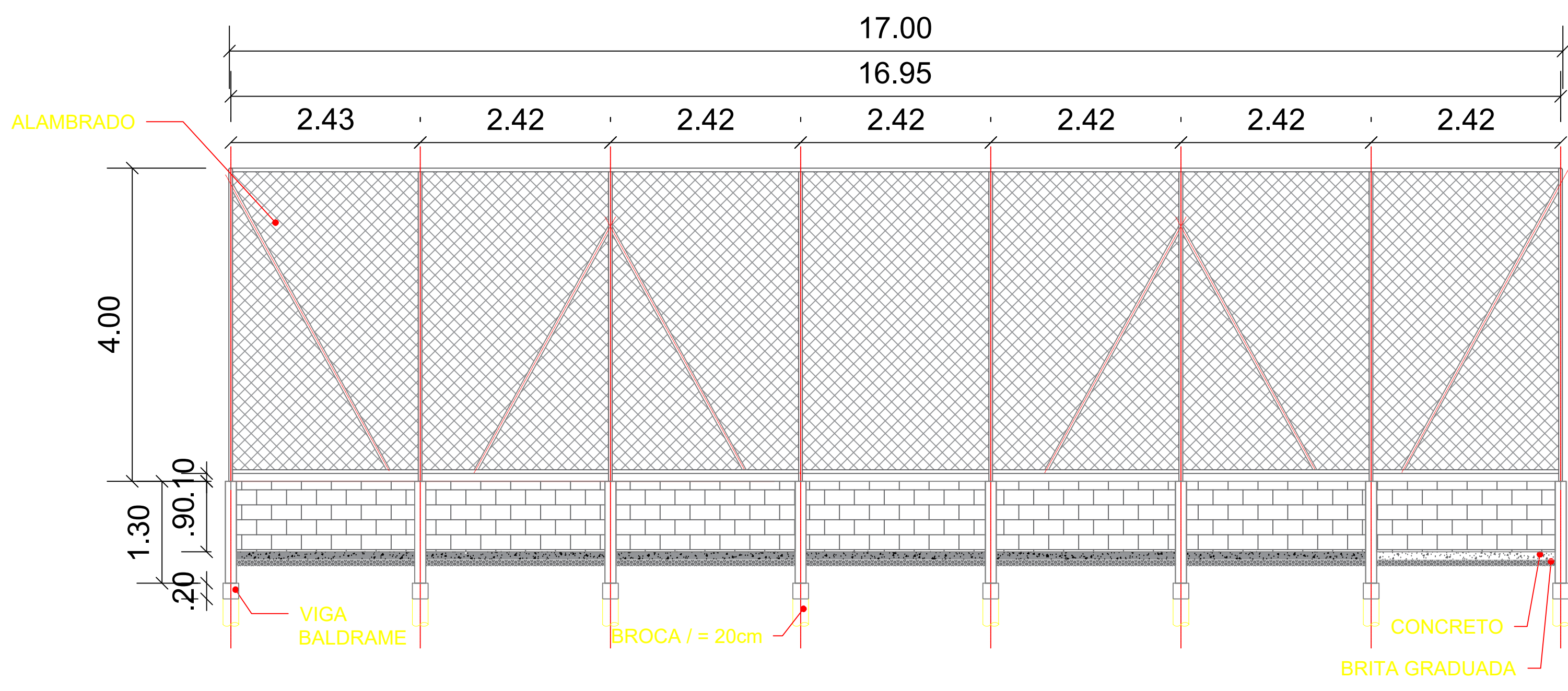
QUADRA POLIESPORTIVA - ELEVÇÃO 02 1:50 03
