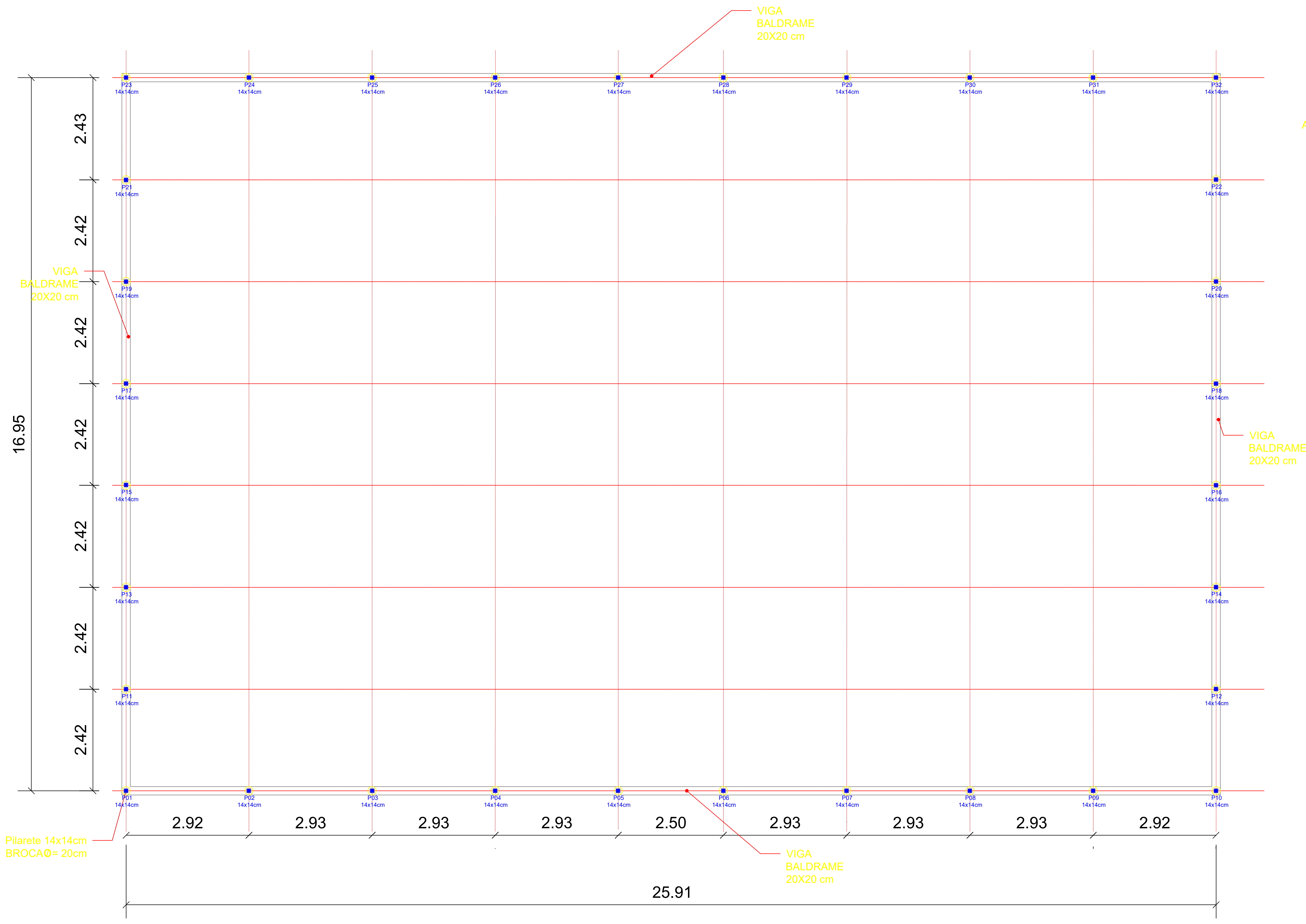
QUADRA POLIESPORTIVA - FUNDAÇÃO 1:50 01
