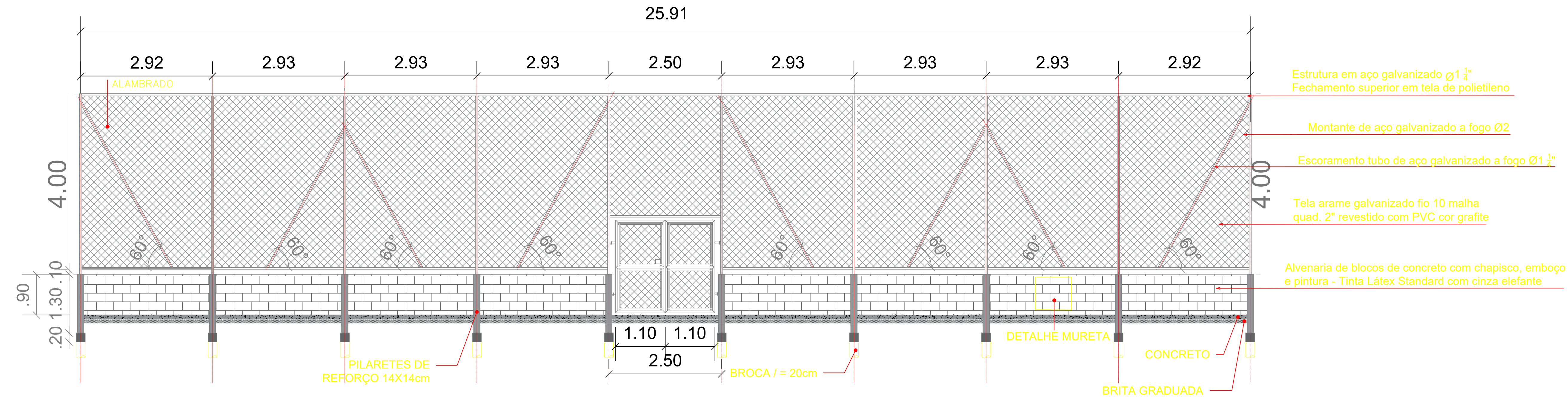
QUADRA POLIESPORTIVA - ELEVÇÃO 01 1:50 02
