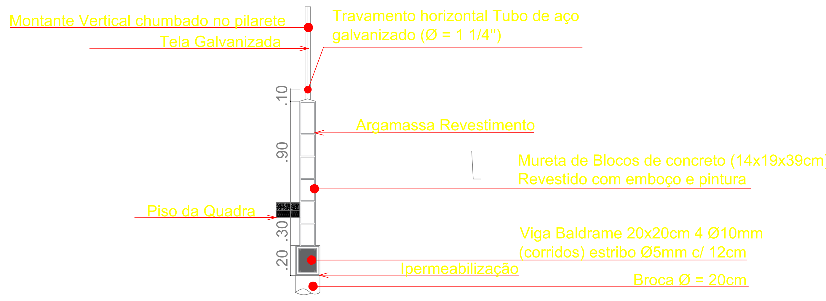
DETALHAMENTO MURETA 1:20 04
