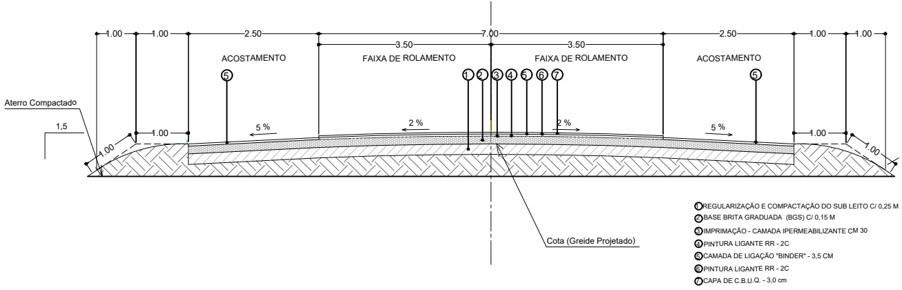
SEÇÃO TRANSVERSAL DO PAVIMENTO - A_A Escala 1:100
