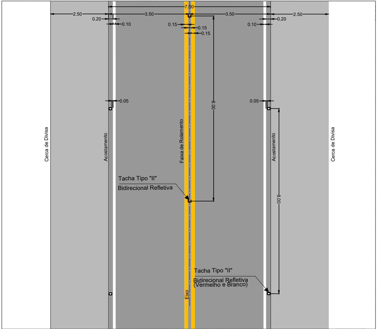
DETALHE "A" Escala 1:100
