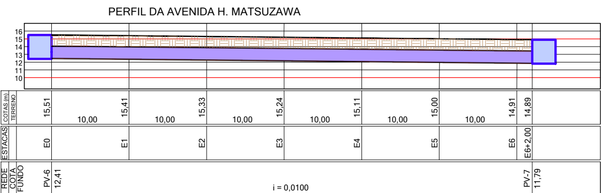
PERFIL 1000 X 1000 ESC. 1:500
