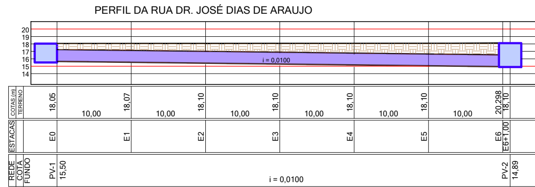
PERFIL 1000 X 1000 ESC. 1:500
