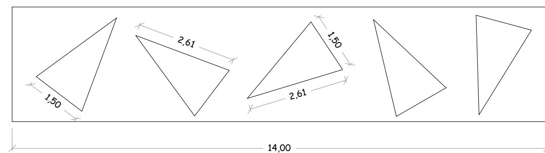
DETALHE 02- Esc. 1:100 (MURO)
