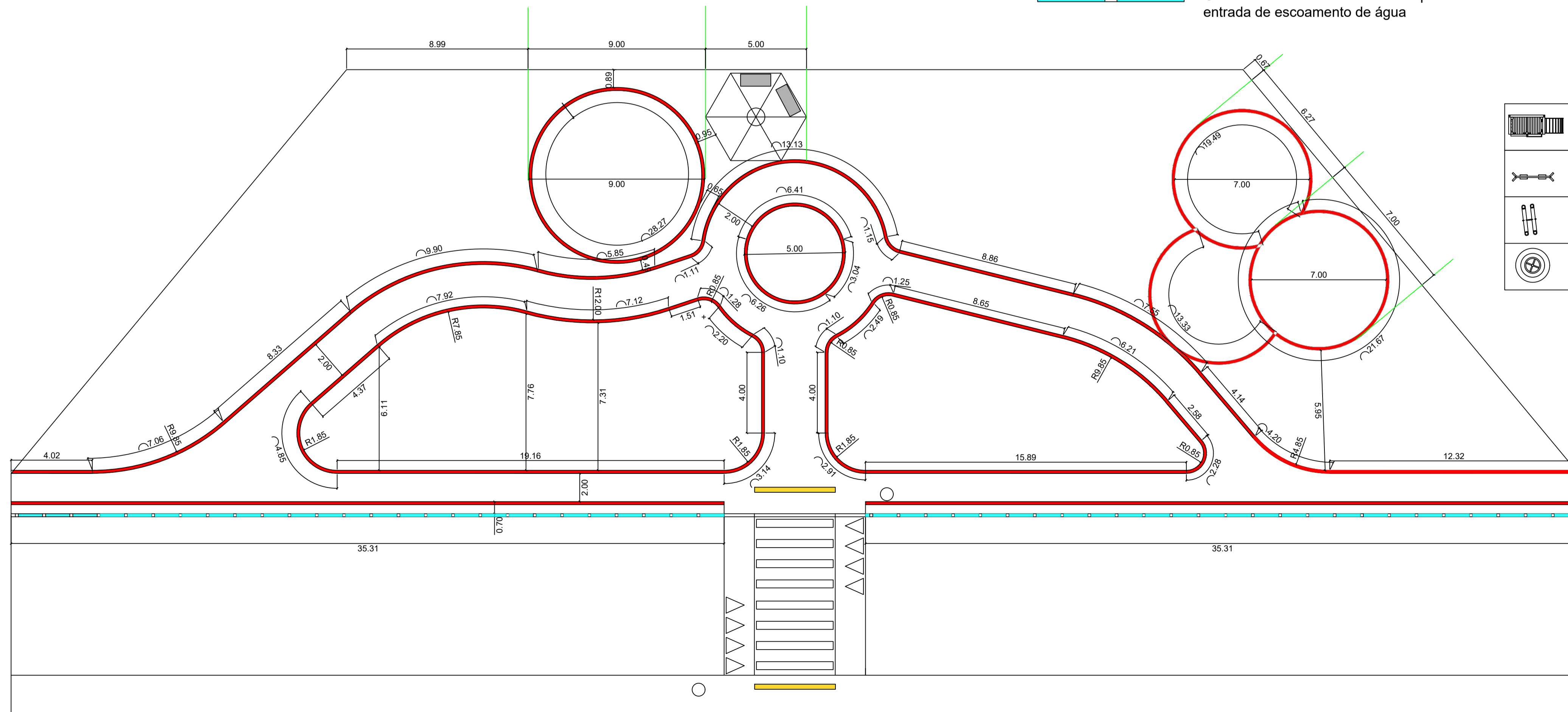
DEMARCAÇÃO DE GUIAS PARA EXECUÇÃO DO CALÇAMENTO E DELIMITAÇÃO DOS CANTEIROS ESC 1/75
