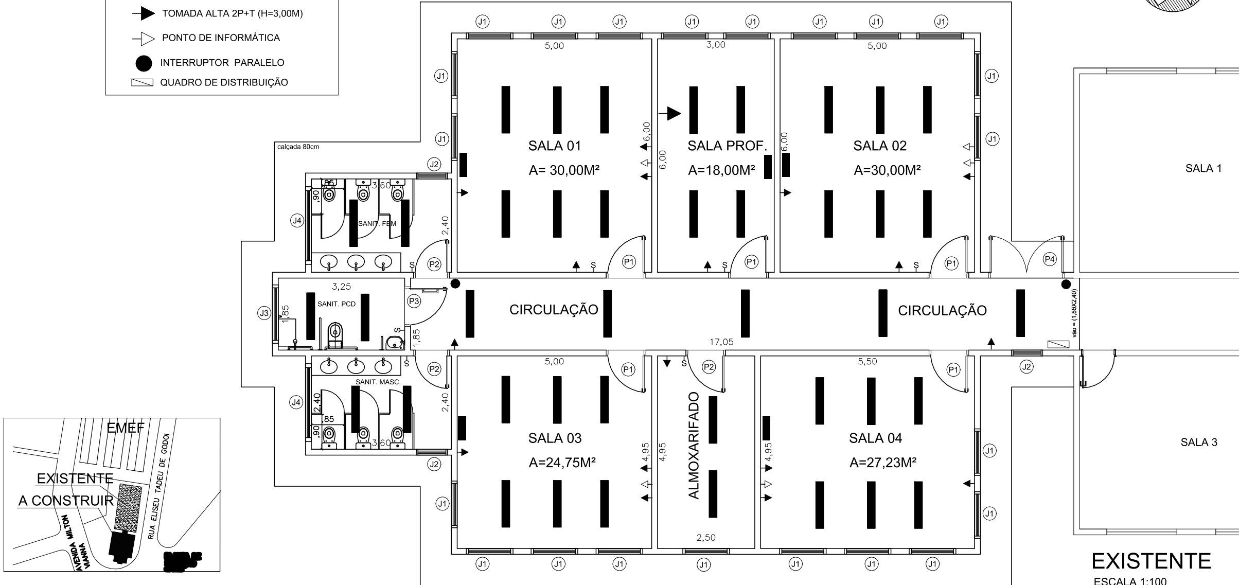
AMPLIAÇÃO ESCALA 1:100
