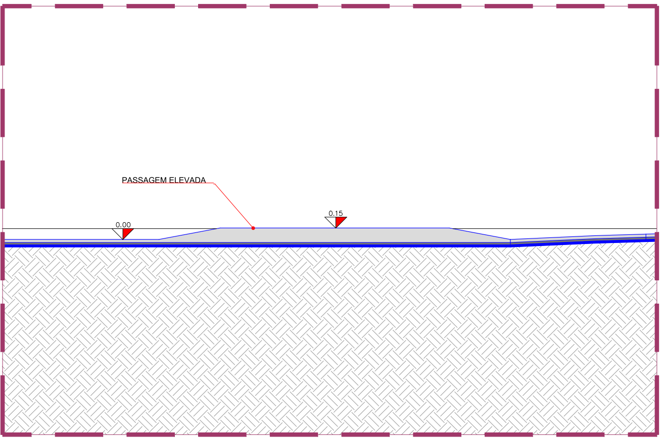
DETALHE 1 - PASSAGEM ELEVADA ESC. 1:50
