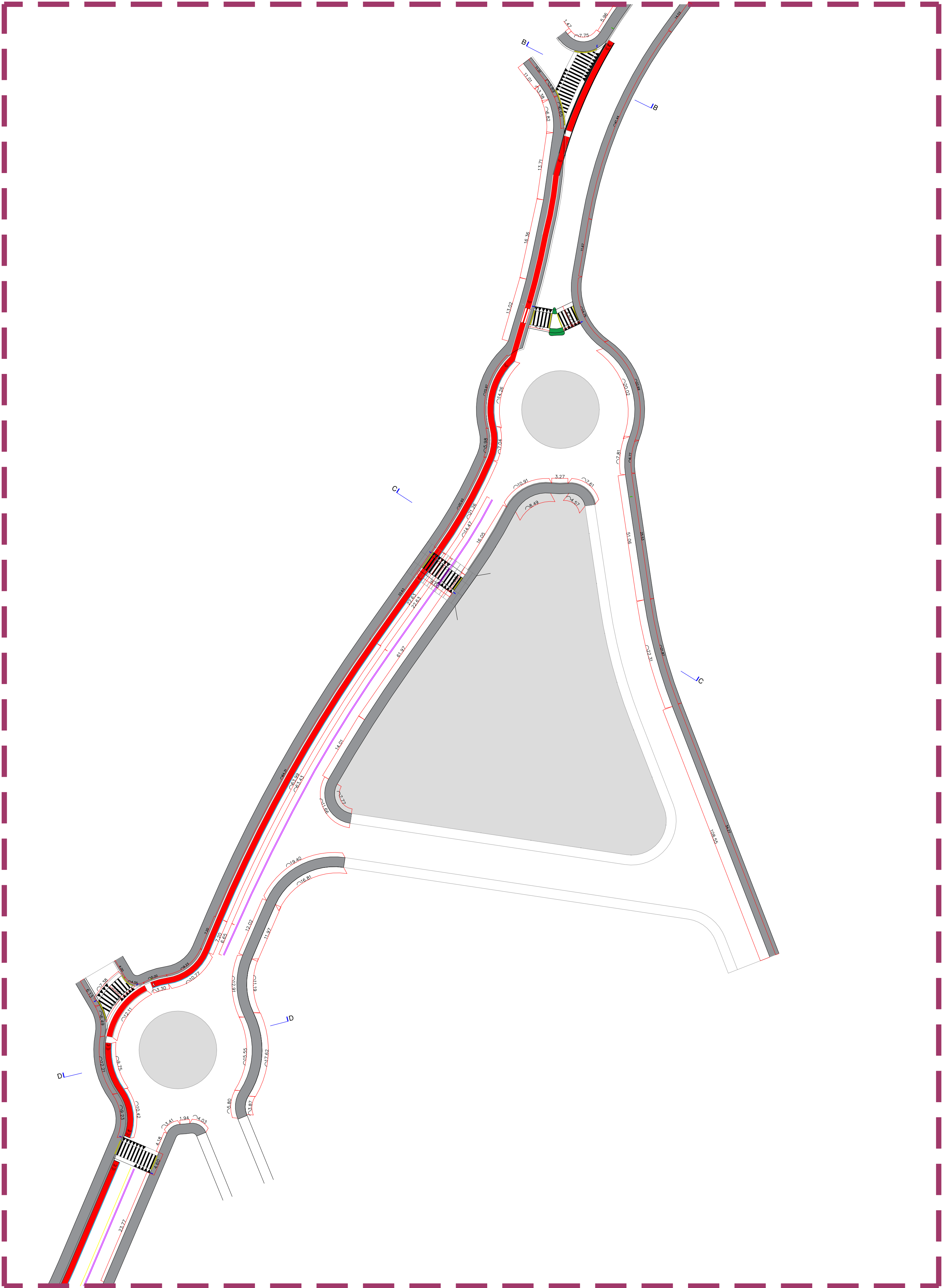
IMPLANTAÇÃO TRECHO 01
