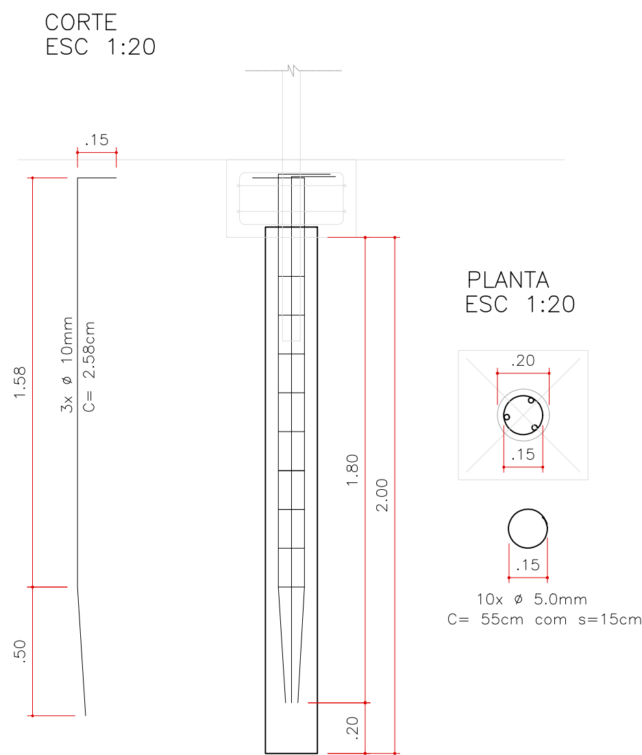
0 DETALHAMENTO ESTACAS ESCALA 1:20
