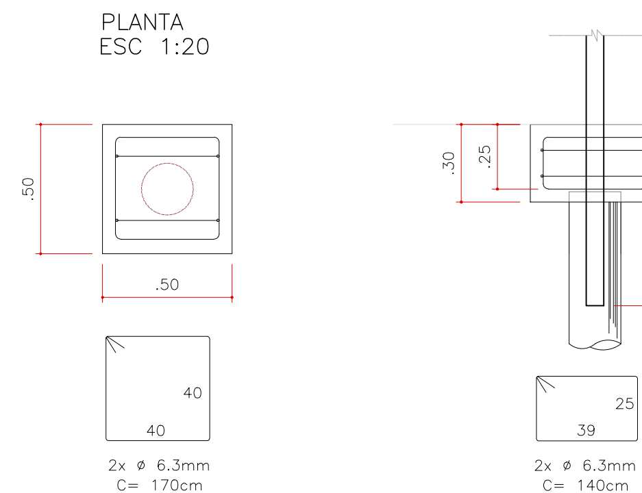
0 DETALHAMENTO BLOCO DE FUNDAÇÃO ESCALA 1:20
