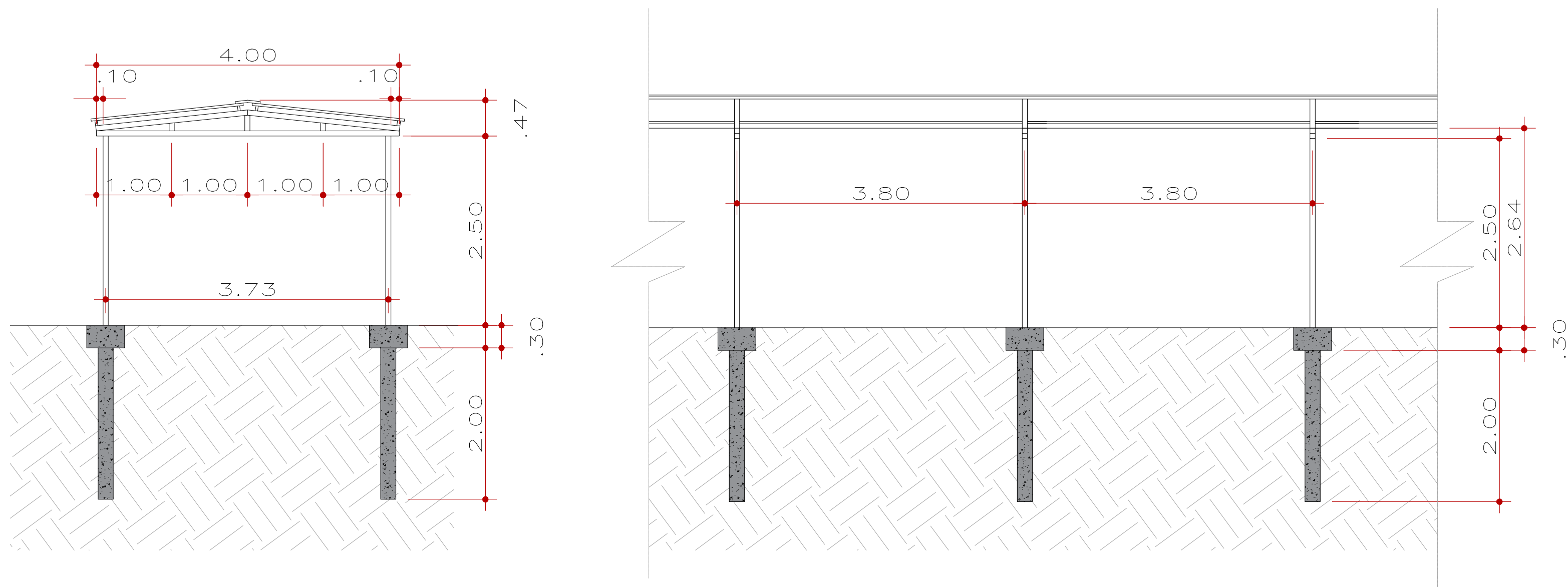
0 DETALHAMENTO DO COBERTURA 03 ESCALA 1:50
