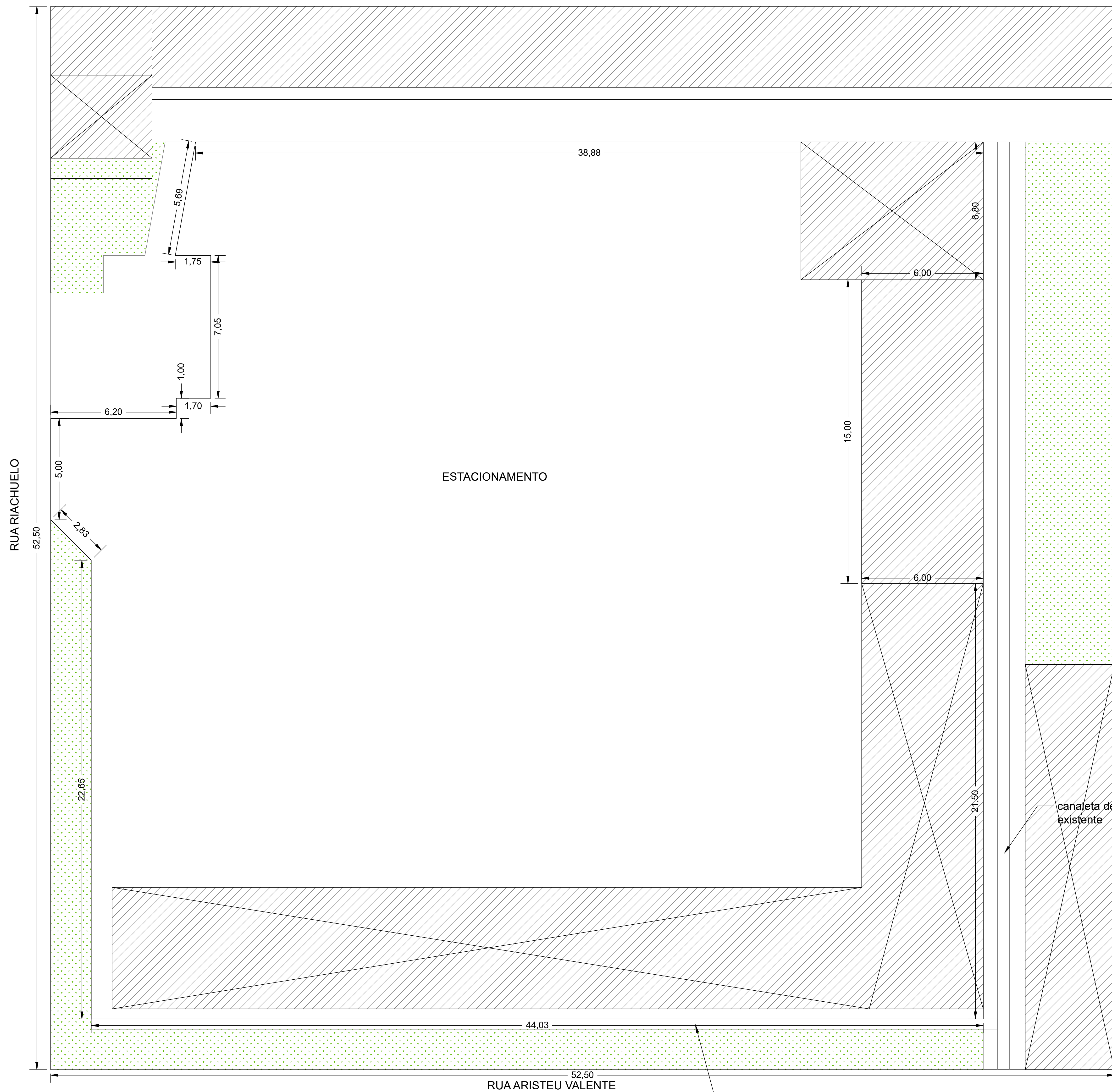
PLANTA BAIXA - ESTACIONAMENTO SETOR DE TRÂNSITO ESCALA 1:250
