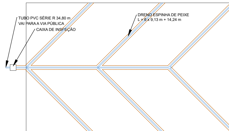
SISTEMA DE DRENAGEM - QUADRA DE VÔLEI ESCALA 1:250
