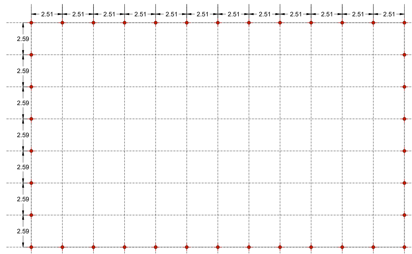
PLANTA DE LOCAÇÃO DAS ESTACAS - QUADRA SOCIETY ESCALA 1:250
