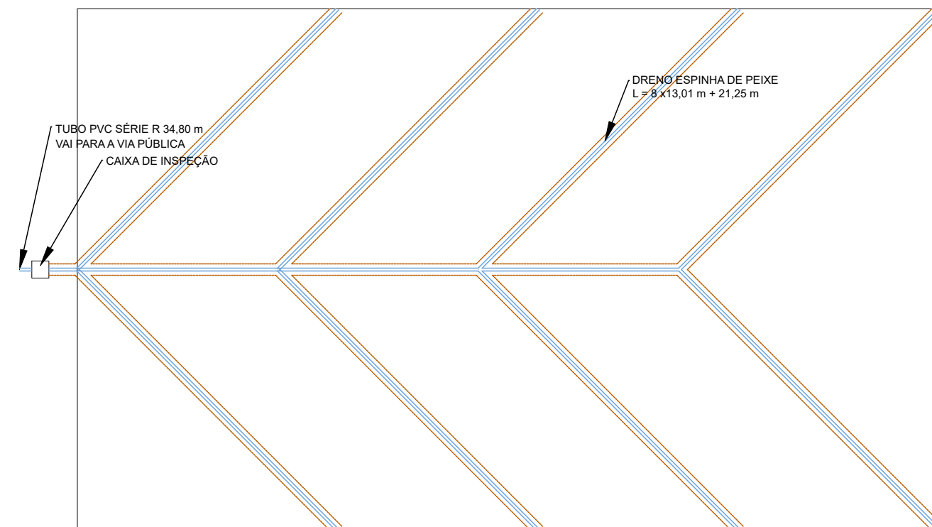
SISTEMA DE DRENAGEM - QUADRA SOCIETY ESCALA 1:250
