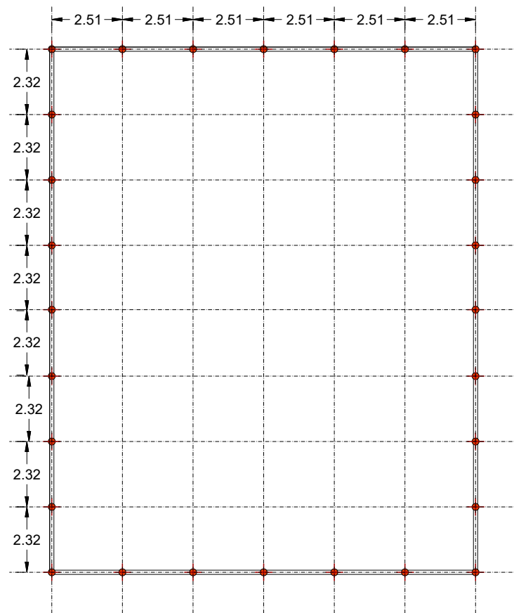
LOCAÇÃO DE ESTACAS - QUADRA DE BASQUETE ESCALA 1:250
