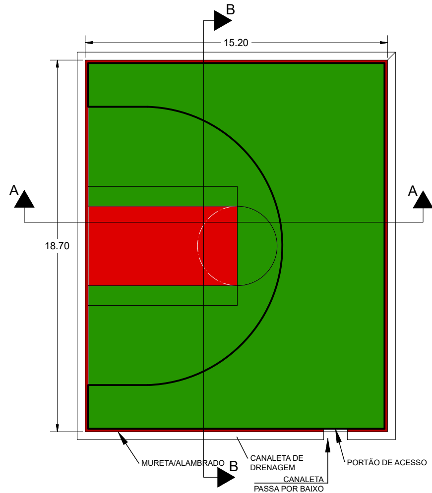
PLANTA BAIXA - QUADRA DE BASQUETE ESCALA 1:250
