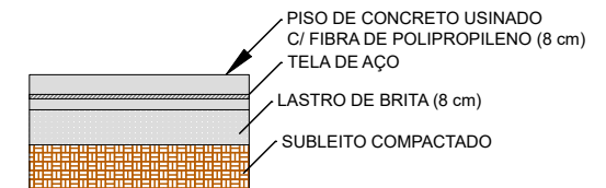
DETALHAMENTO PISO - QUADRA DE BASQUETE ESCALA 1:25
