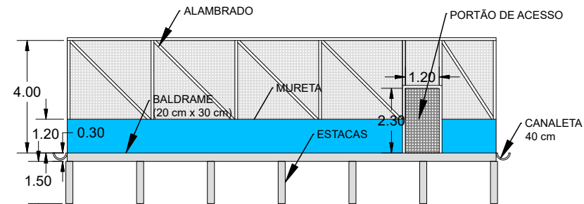
CORTE A-A - QUADRA DE BASQUETE ESCALA 1:250
