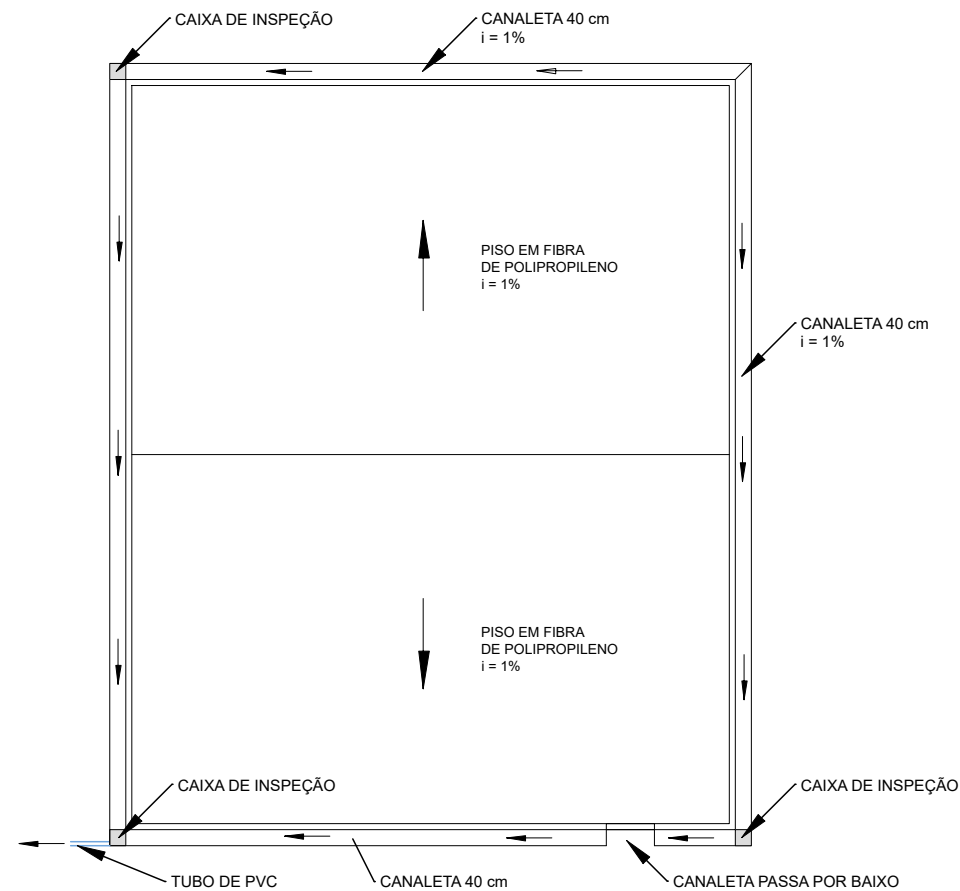
SISTEMA DE DRENAGEM - QUADRA DE BASQUETE ESCALA 1:250
