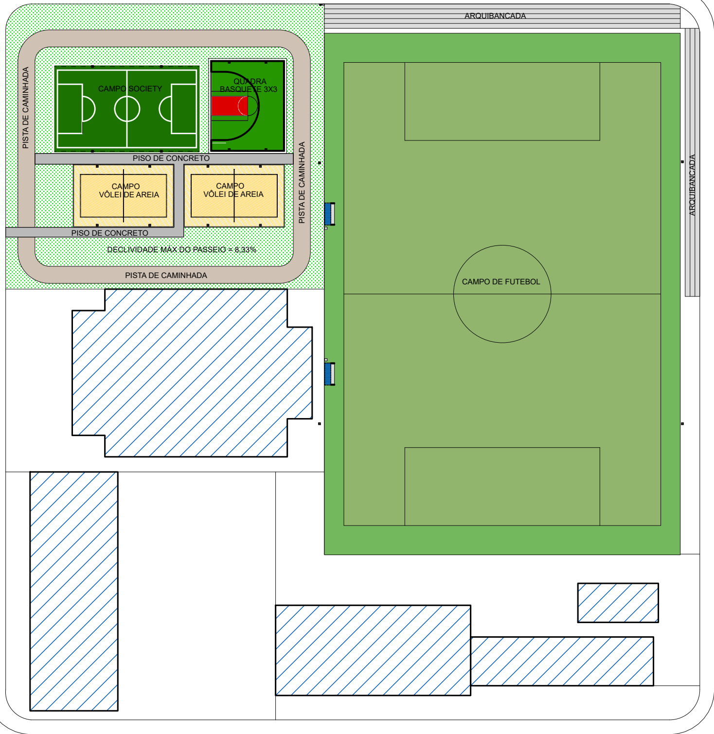
IMPLANTAÇÃO ESCALA 1:1000
