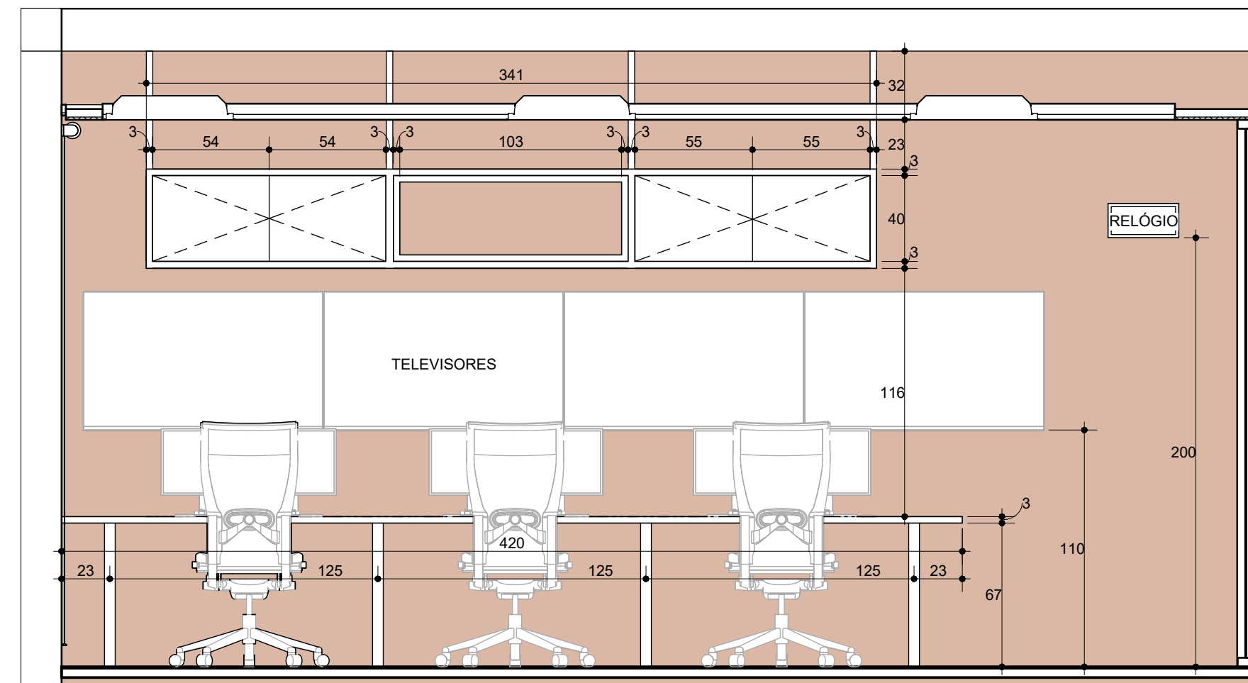
5 VA - 02 1 : 25
