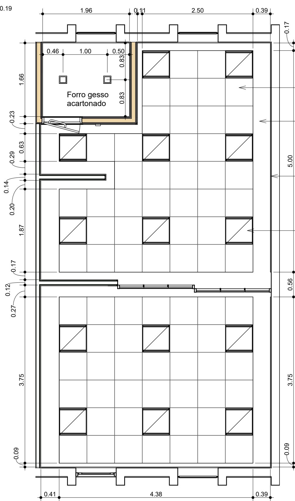
2 Forro e iluminação 1 : 50
