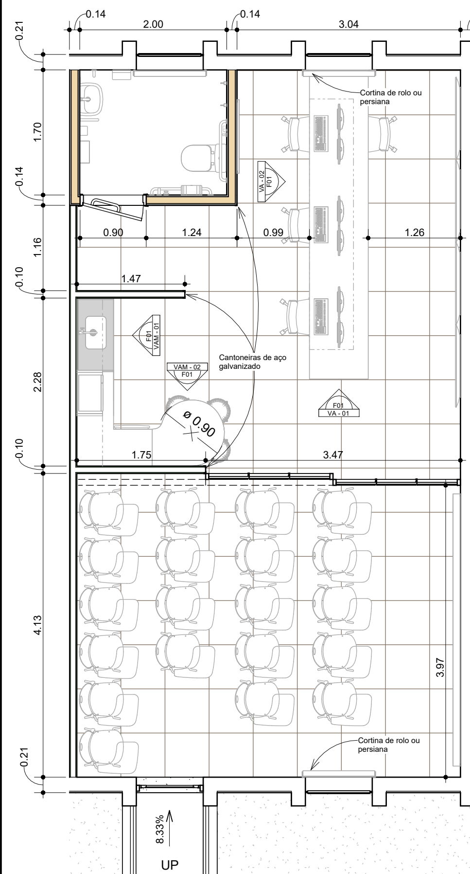
1 Planta e layout 1 : 50
