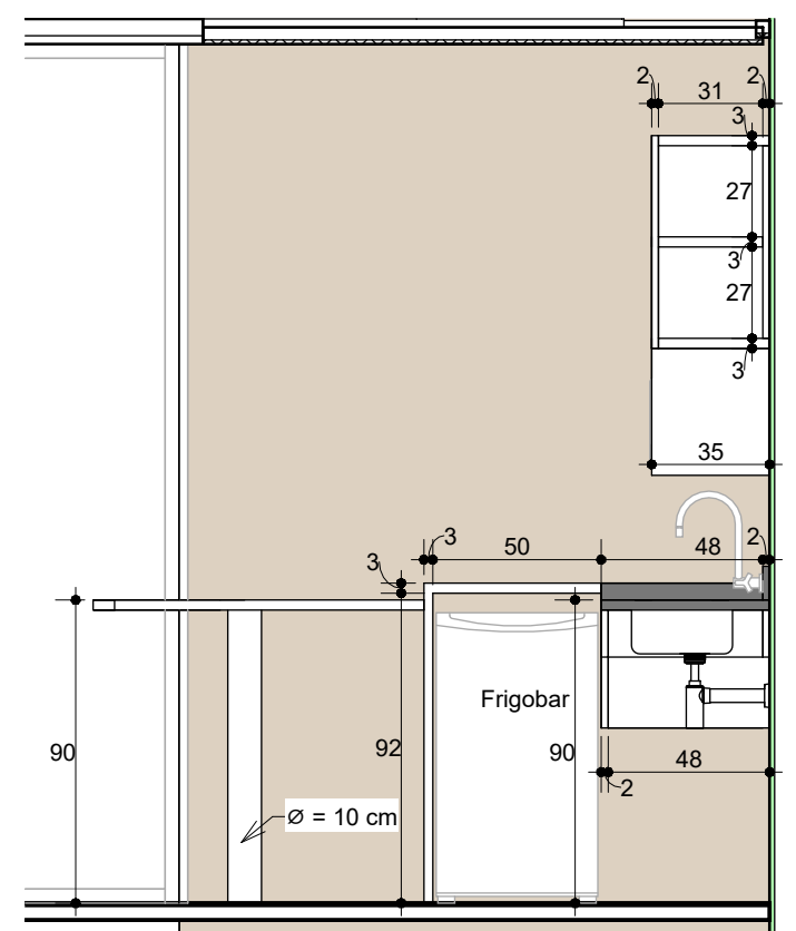
4 VAM - 02 1 : 25
