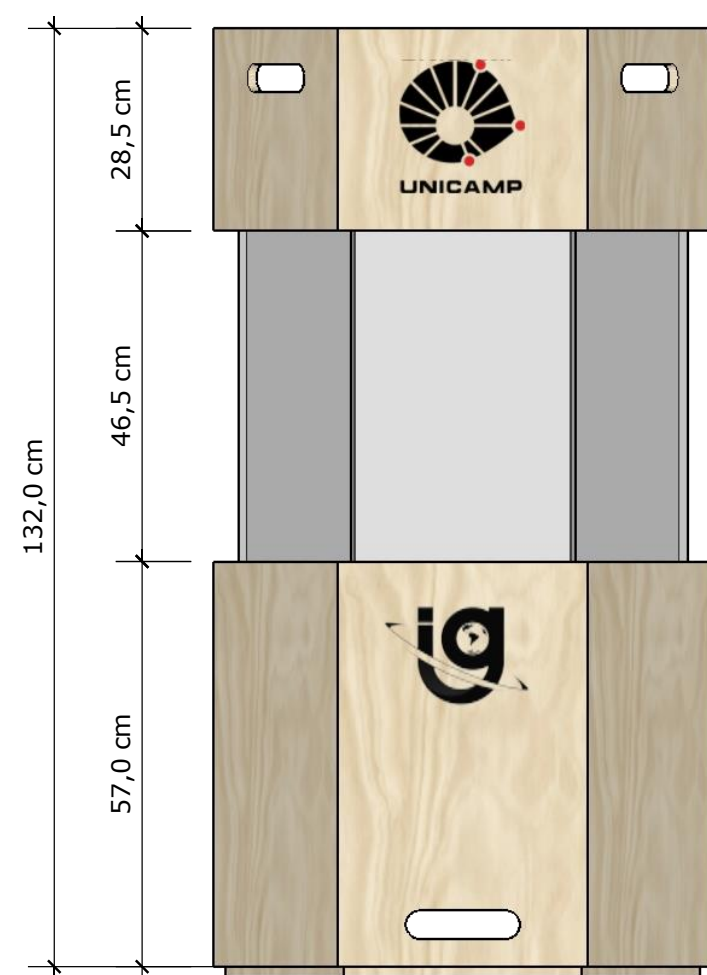
VISTA FRONTAL ESCALA 1:10
