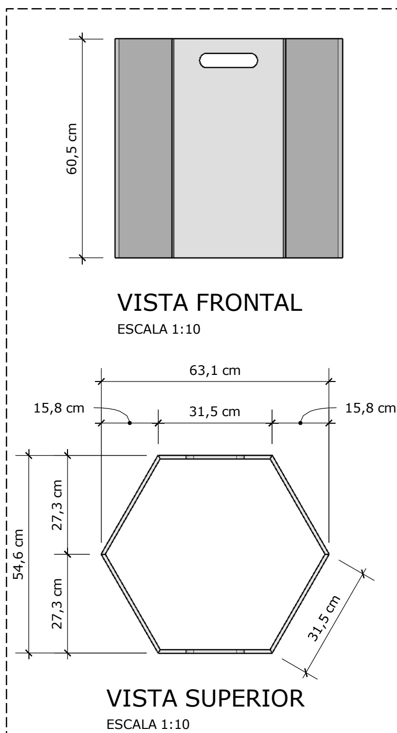
PEÇA C (07 UNID.)
