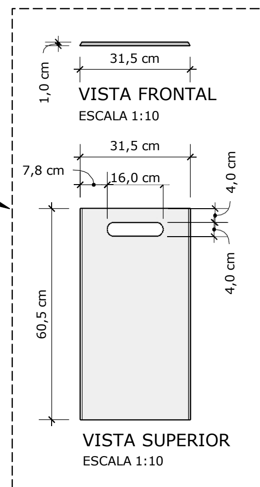
PEÇA F2 (02 UNID.)
