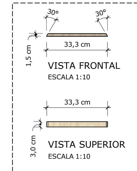
PEÇA D (42 UNID.)
