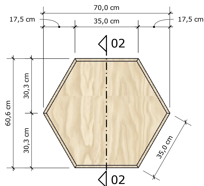
VISTA SUPERIOR ESCALA 1:10
