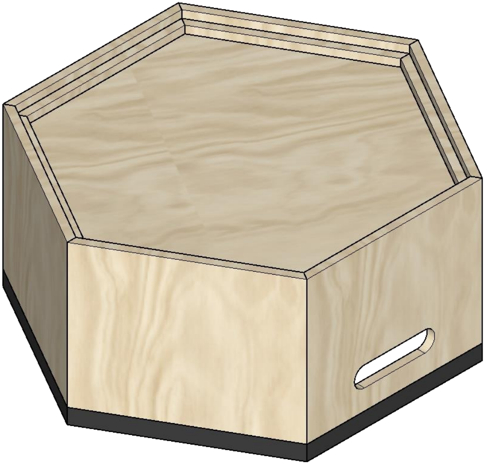
PERSPECTIVA - MÓDULO BASE ESCALA 1:5
