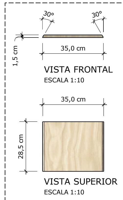
PEÇA A1 (18 UNID.)
