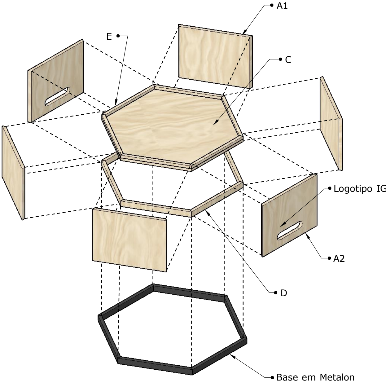
PERSPECTIVA EXPLODIDA ESCALA 1:10
