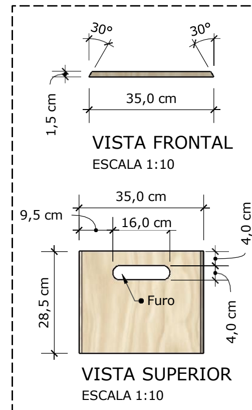
PEÇA A2 (12 UNID.)
