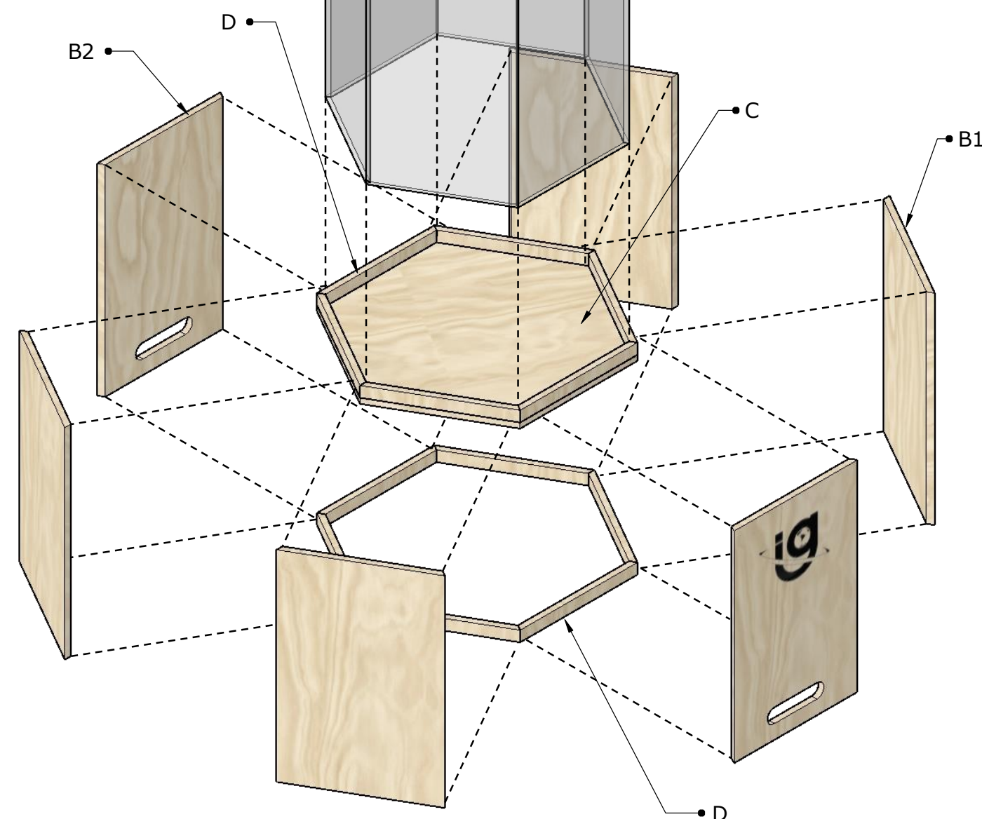
PERSPECTIVA EXPLODIDA ESCALA 1:10
