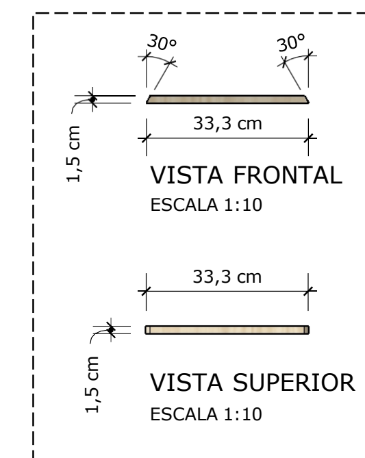
PEÇA E (30 UNID.)
