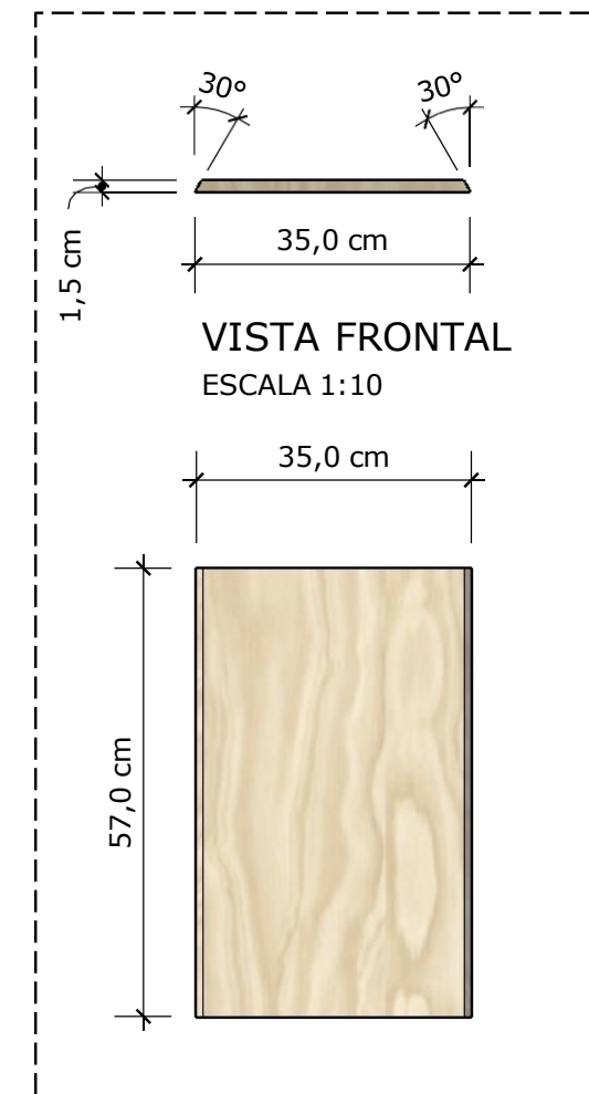
PEÇA B1 (04 UNID.)
