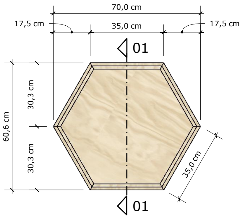
VISTA SUPERIOR ESCALA 1:10
