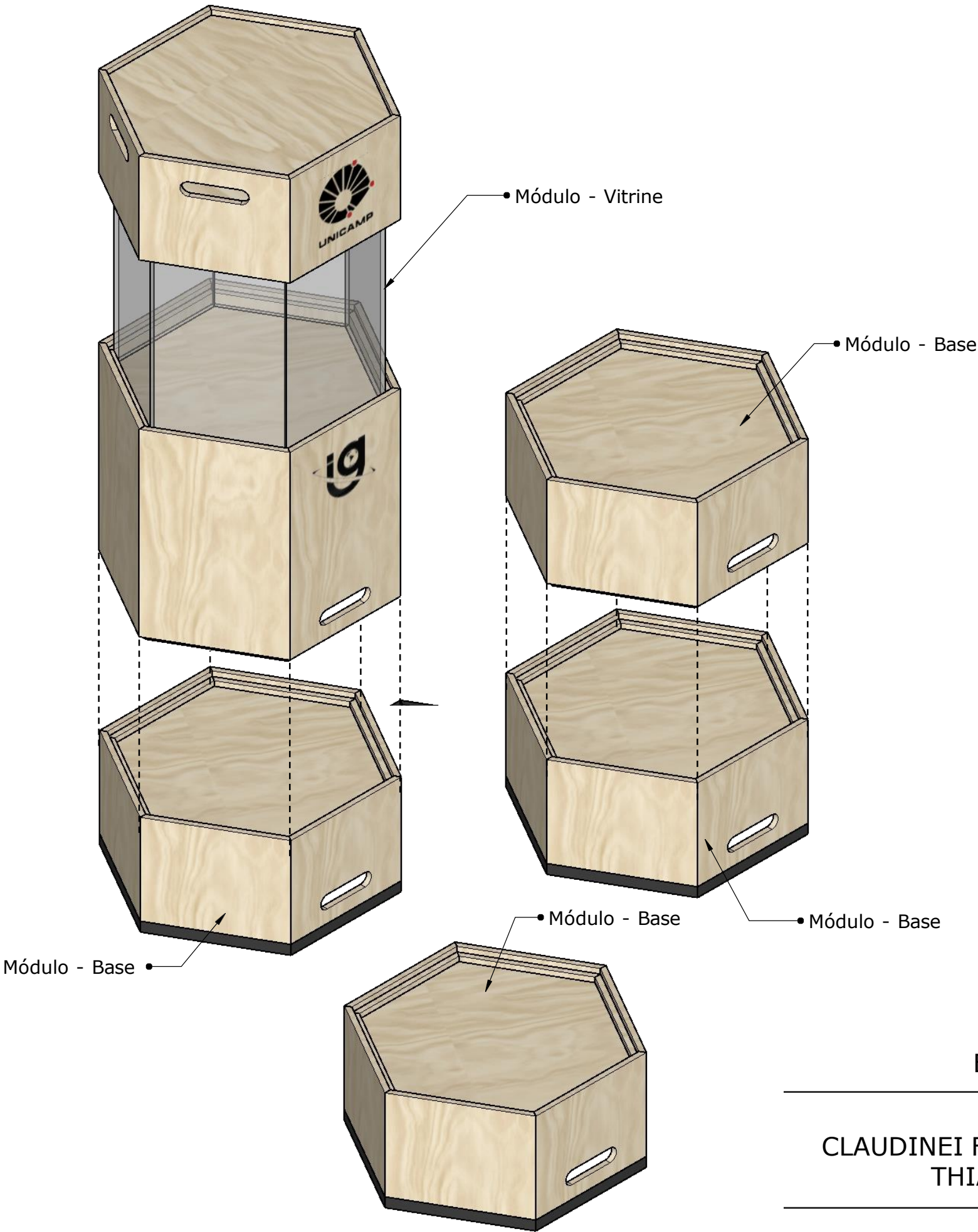
PERSPECTIVA GERAL - MODULAÇÃO ESCALA 1:10
