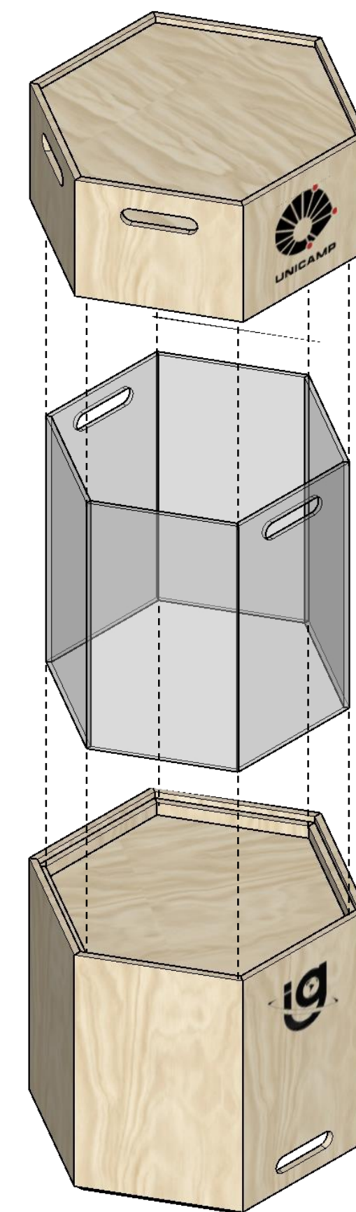
PERSPECTIVA MONTAGEM ESCALA 1:10
