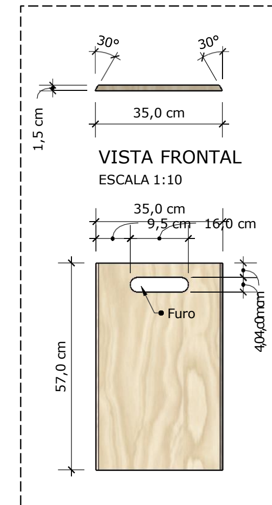
PEÇA B2 (02 UNID.)
