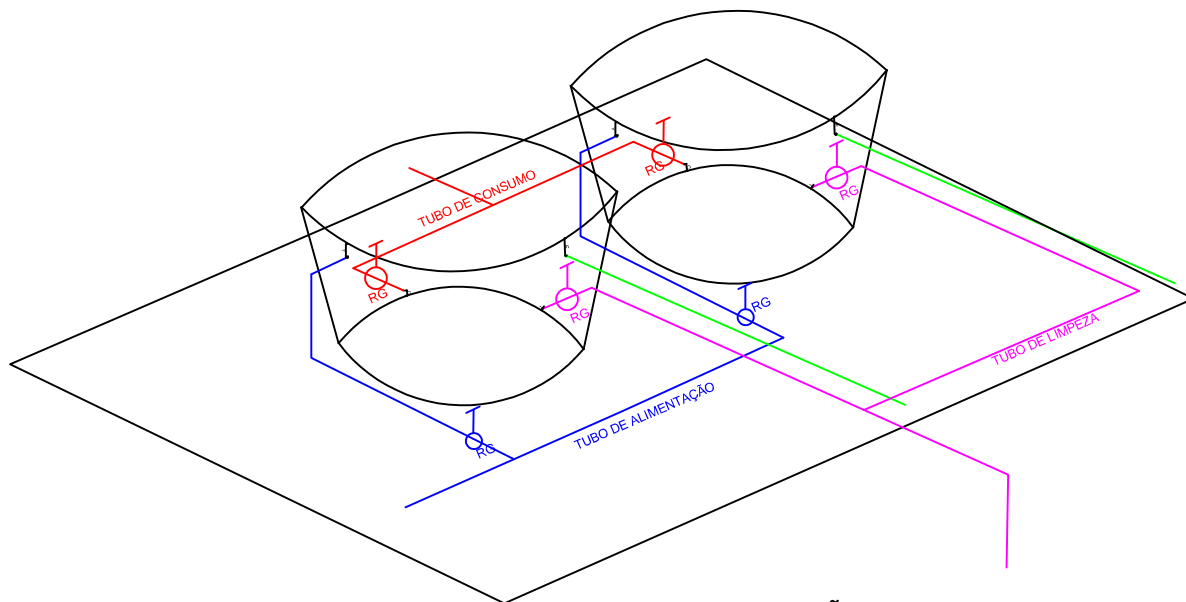
DETALHE DAS TUBULAÇÕES
