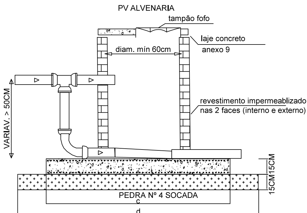
RELAÇÃO PROFUNDIDADE X DIÂMETRO PV
