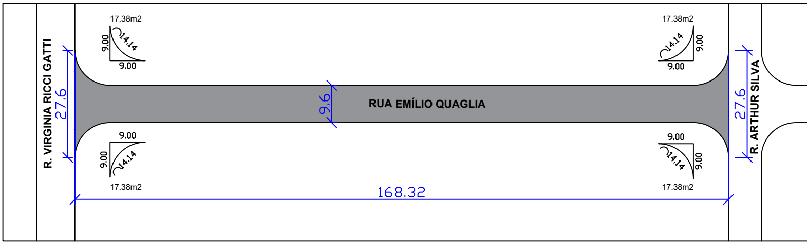
RECAPEAMENTO ASFALTICO - RUA EMÍLIO QUAGLIA: ÁREA = 1.685,39 m²
