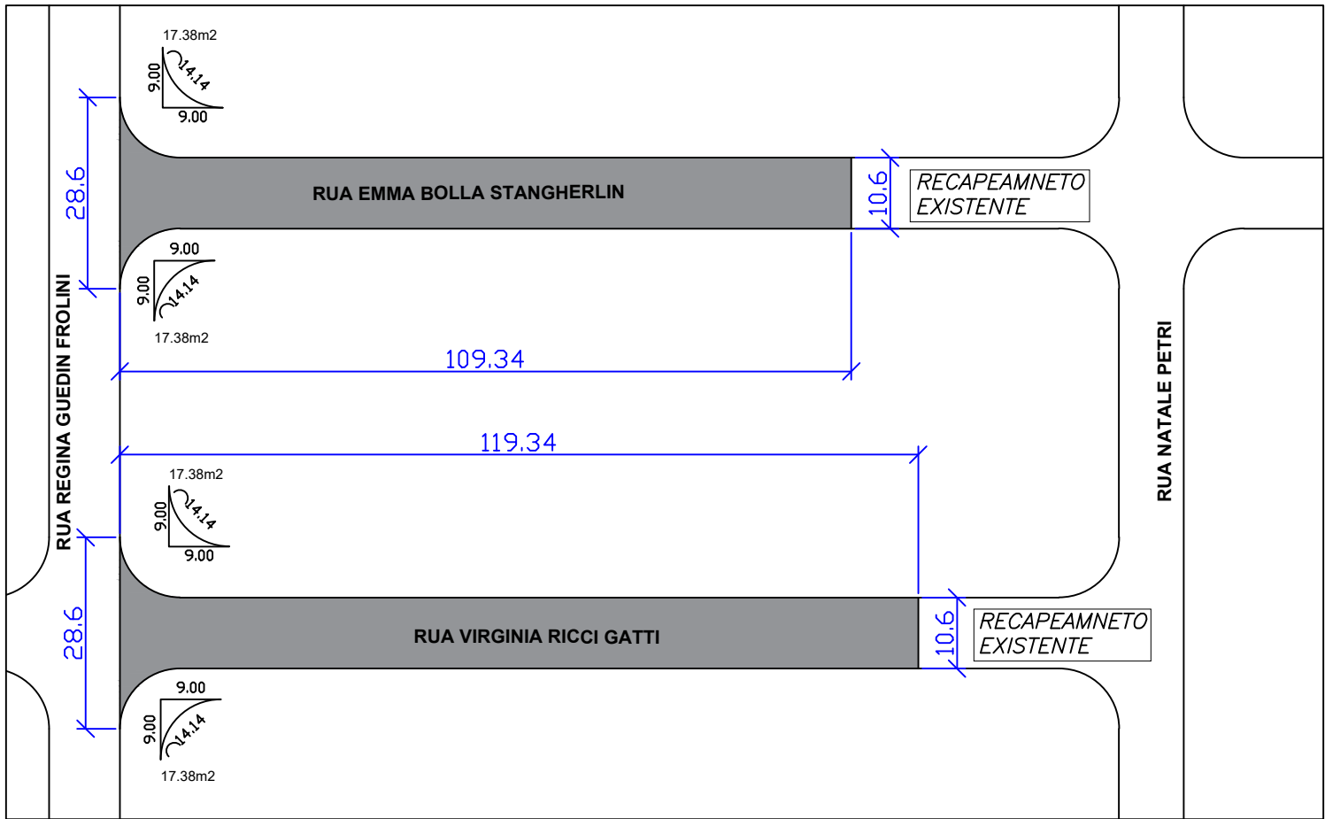
RECAPEAMENTO ASFALTICO - RUA EMMA BOLLA STANGHERLIN: ÁREA = 1.193,76 m² / RUA VIRGINIA RICCI GATTI: ÁREA = 1.299,76 m²
