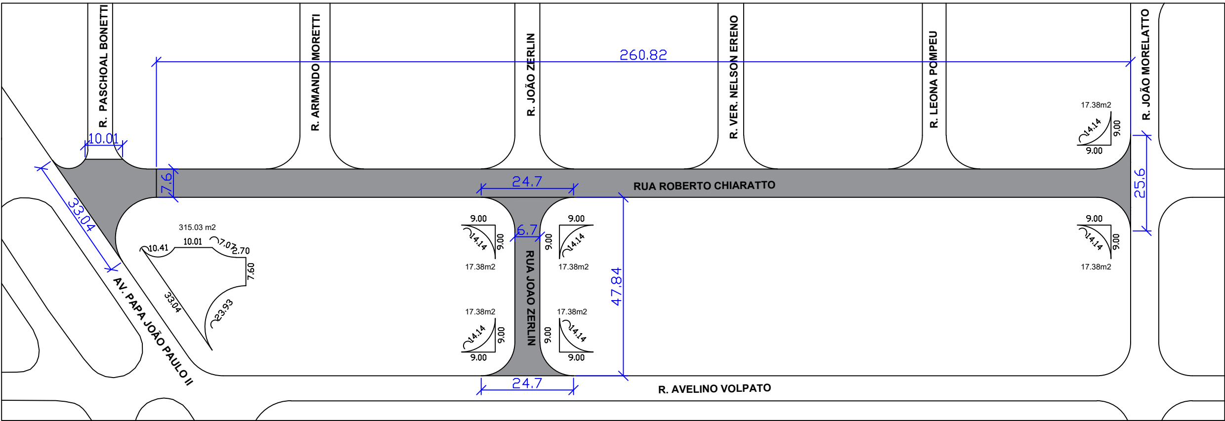
RECAPEAMENTO ASFALTICO - RUA ROBERTO CHIARATTO: ÁREA = 2.332,02 m² / RUA JOAO ZERLIN: ÁREA = 390,05 m²
